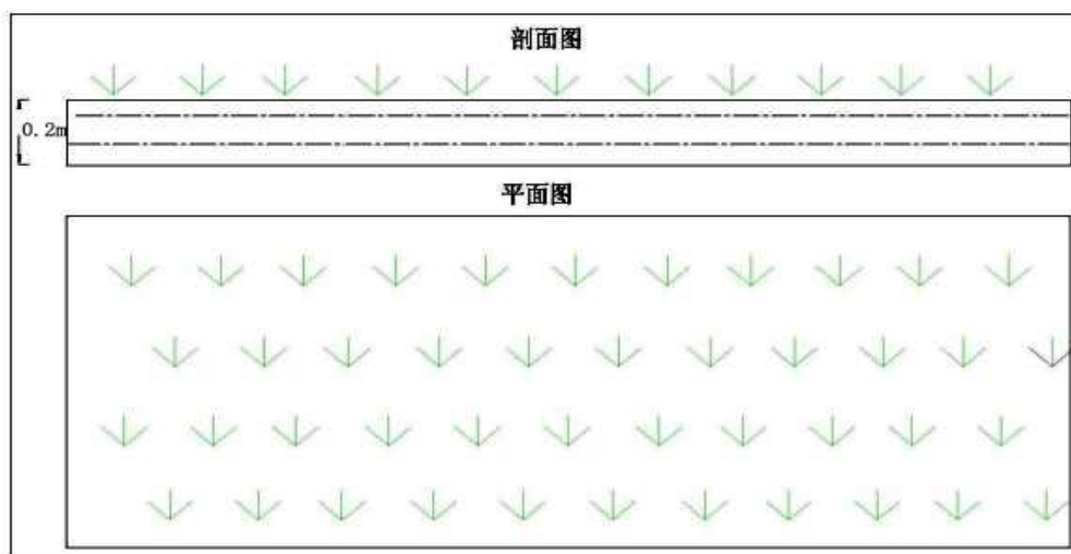
图 5-3 植被恢复示意图
