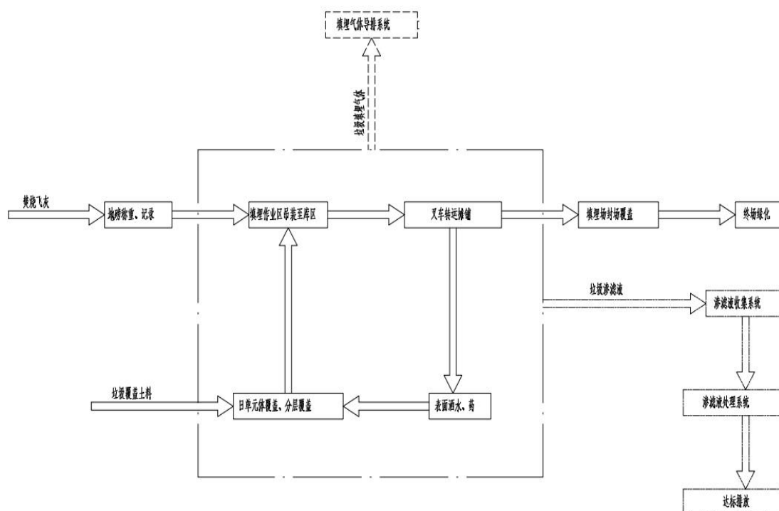
图 5.1-2 填埋工艺流程图
