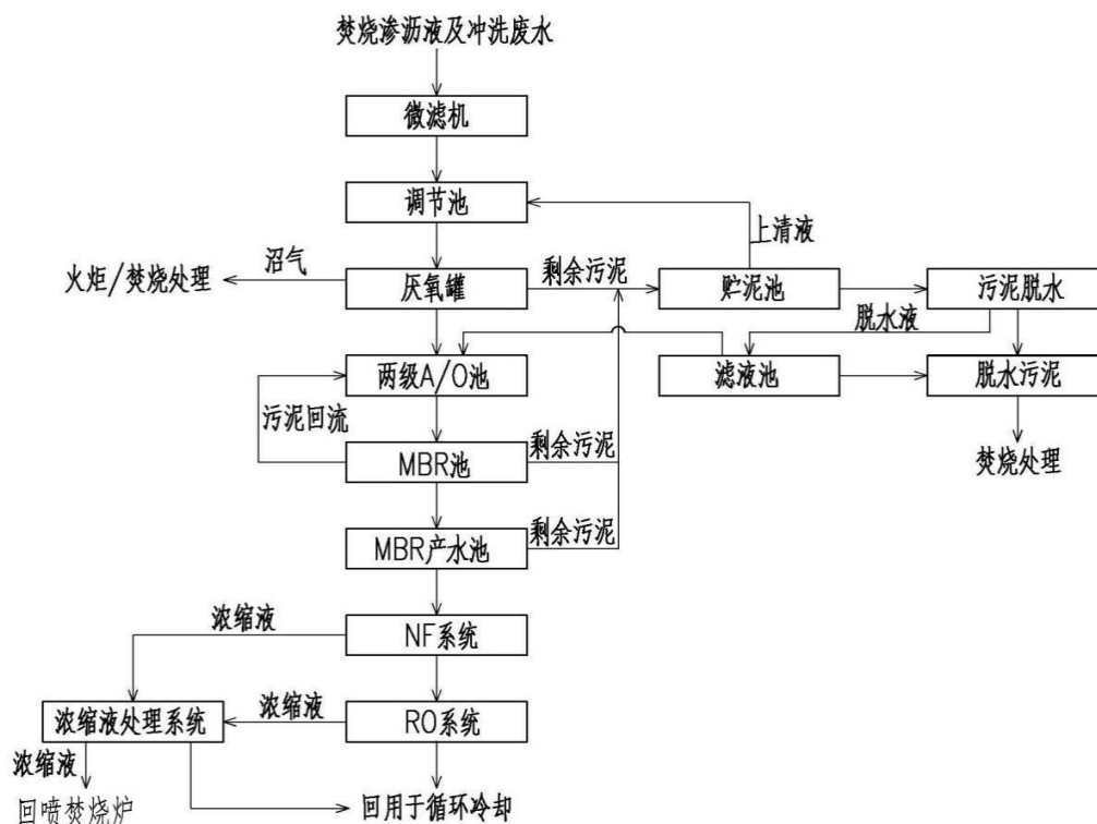
图 8.2-3 生活垃圾焚烧项目渗滤液处理工艺流程图
