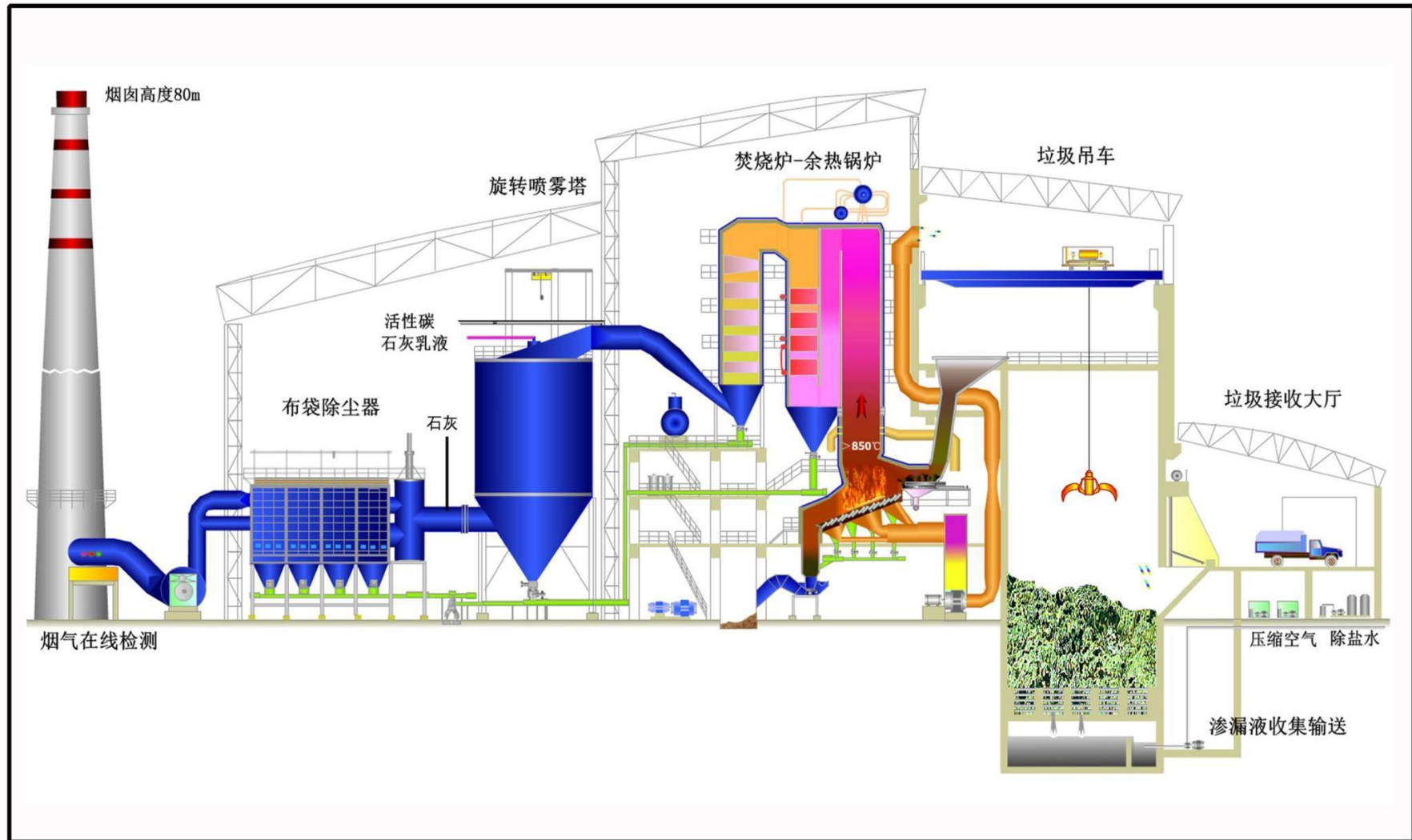
图 3.2-2 生活垃圾焚烧处理工艺流程
