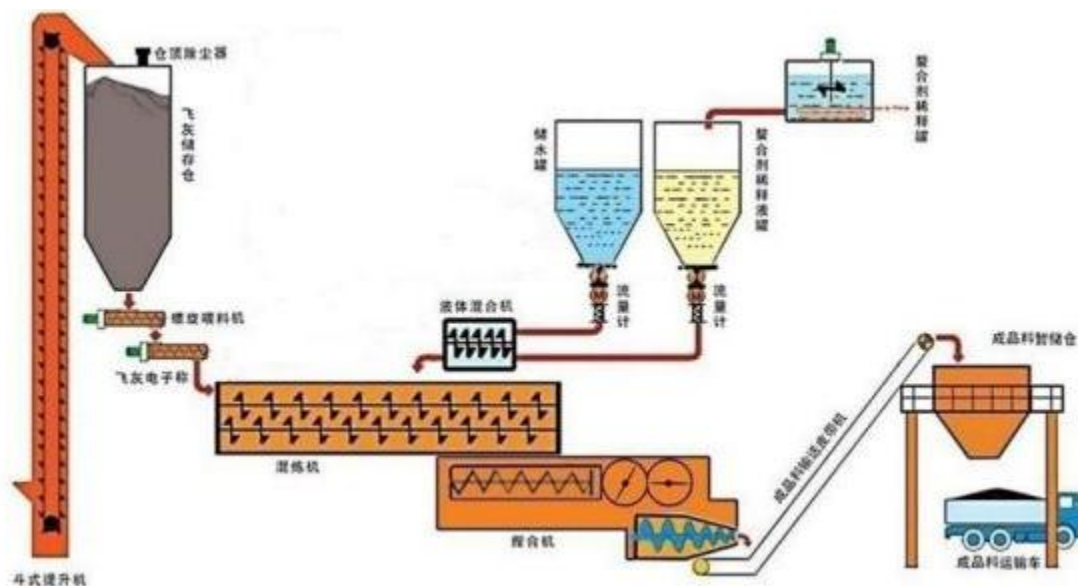
图 3.2-3 飞灰固化工艺流程
