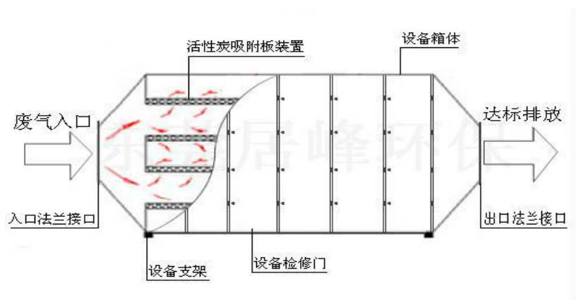
图 3.2-3 活性炭吸附装置示意图
