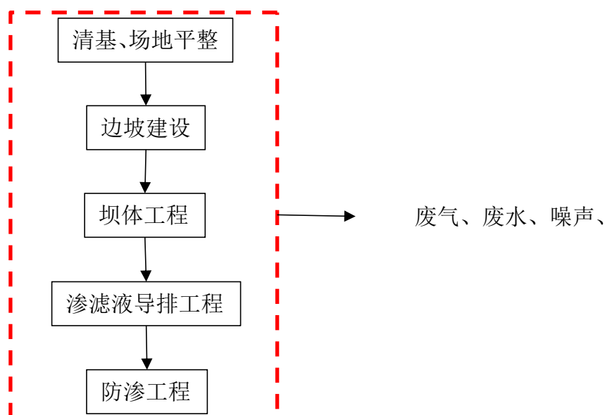
图 5.1-1 施工期工艺流程及产排污节点图
