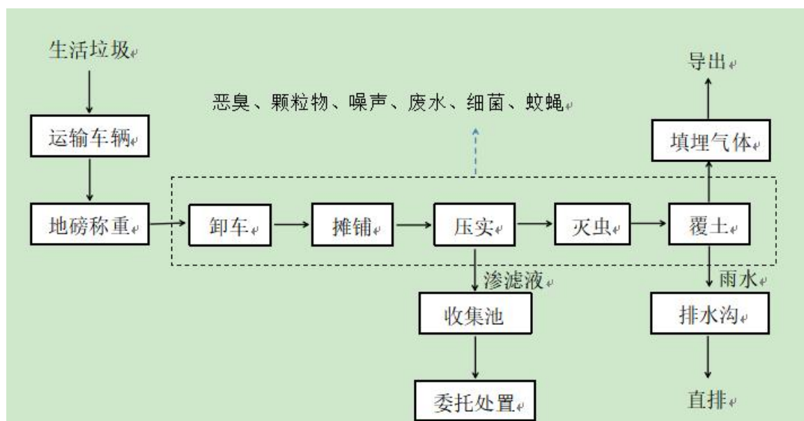
图 3.1-1 填埋工艺流程及产污环节图
