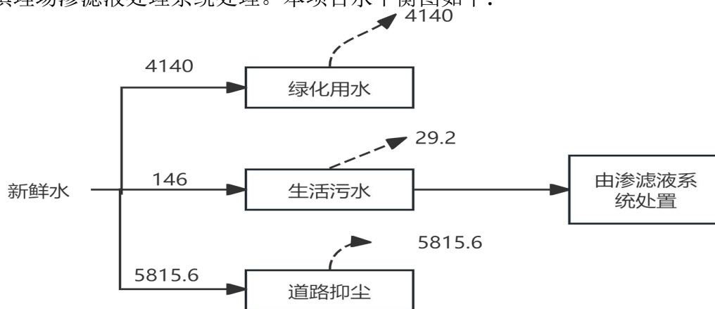
图 4.7-1 水平衡图 单位 t/a
