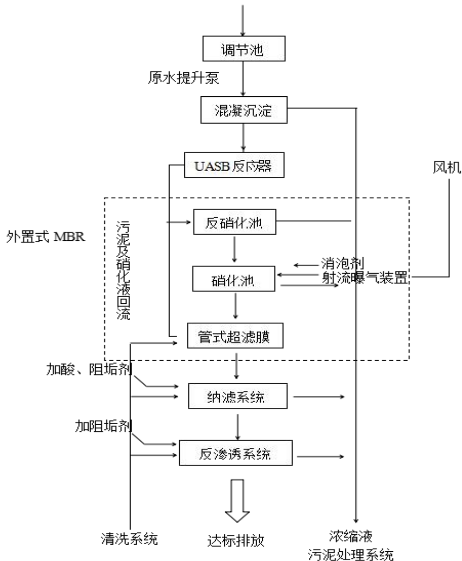
图 8.2-1 50m³/d 的渗滤液处理站处理工艺
