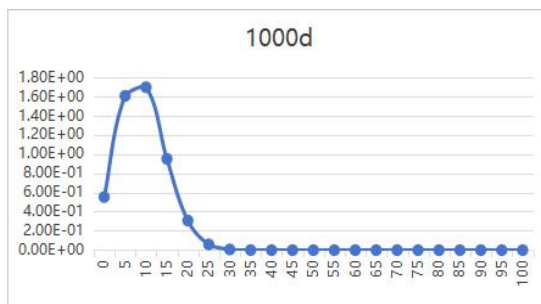
图 7.3-2 1000d, COD 运移浓度分布图
