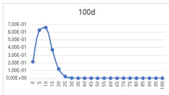
图 7.3-3 100d, NH3-N 运移浓度分布图
