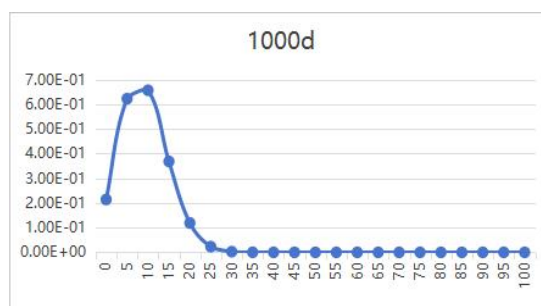
图 7.3-4 1000d, NH3-N 运移浓度分布图
