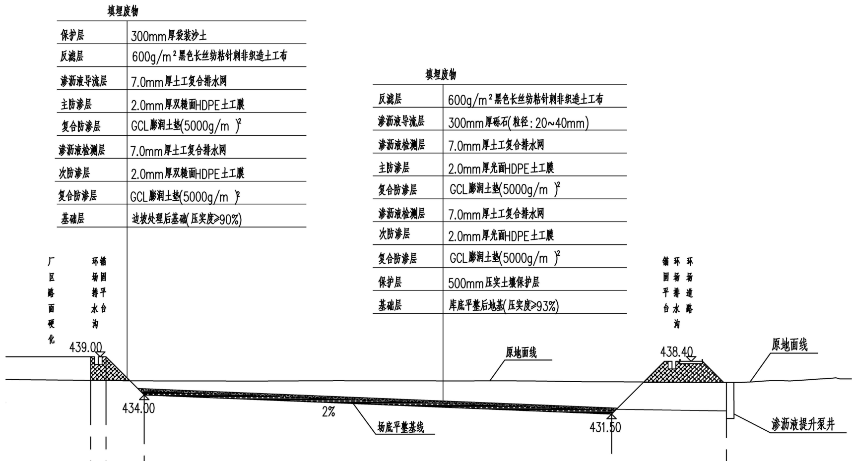
附图 4.6-1 防渗结构图
