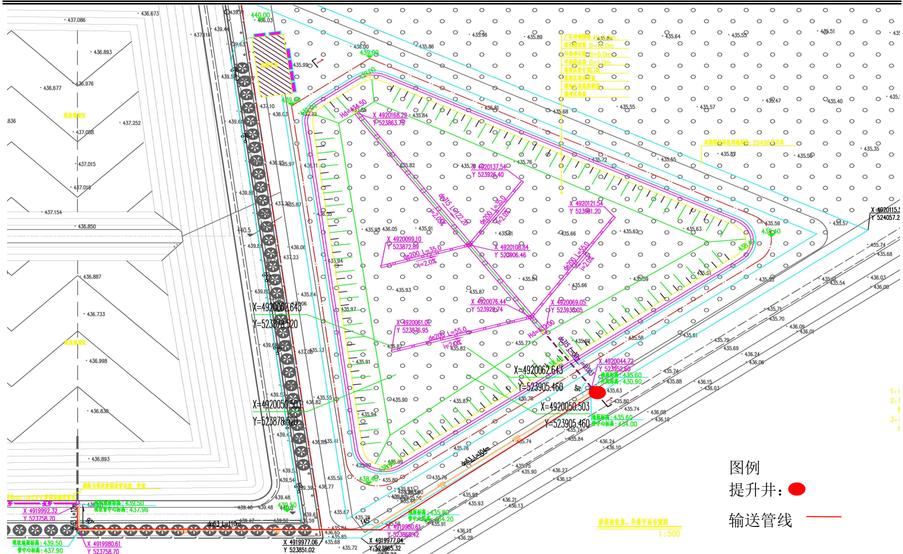
附图 4.6-2 渗滤液收集系统
