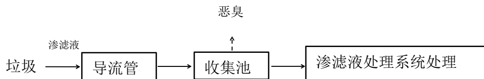
图 3.1-2 渗滤液导排系统及处理工艺流程及产污环节图
