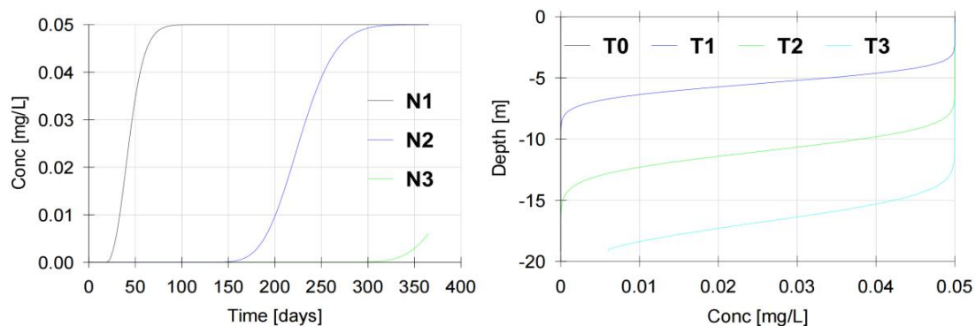
图 7.2-1 土壤中汞浓度变化曲线
