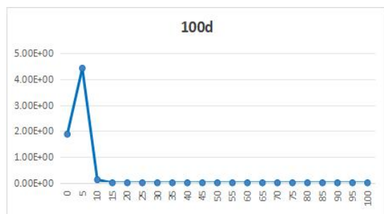
图 7.3-1 100d, COD 运移浓度分布图
