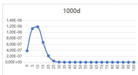
图 7.3-4 1000d, NH3-N 运移浓度分布图
