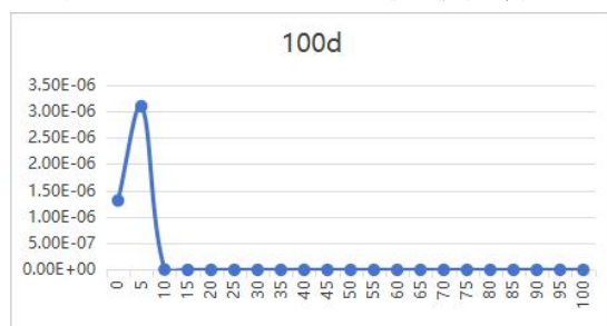
图 7.3-3 100d, NH3-N 运移浓度分布图
