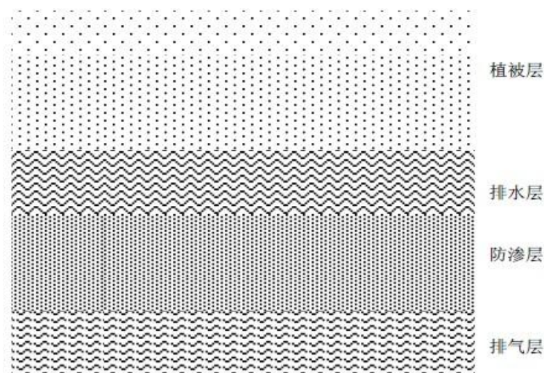
图 8.4-1 封场系统剖面图
