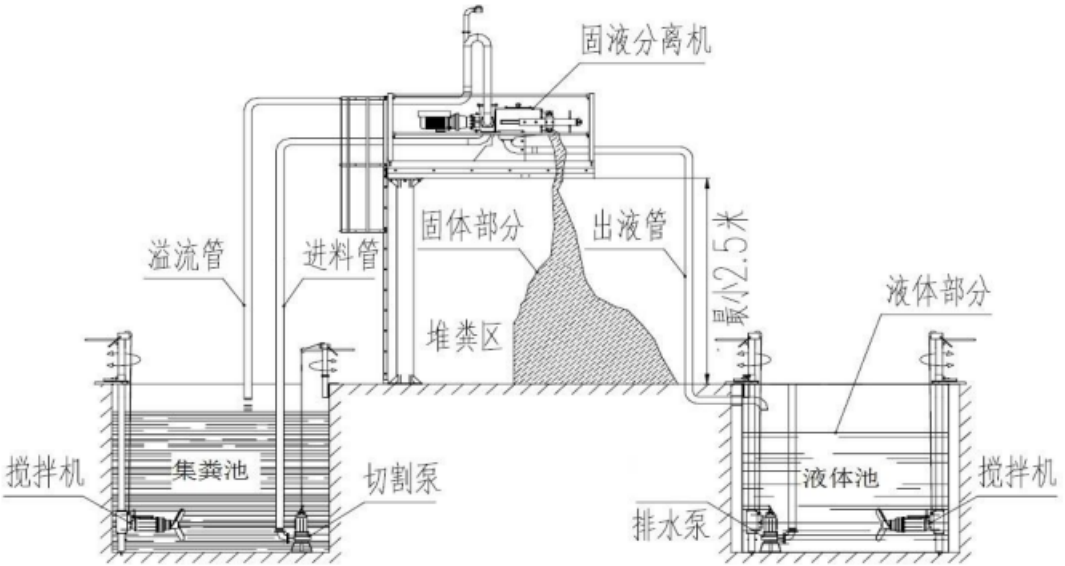
图 4.4-4 固液分离系统断面示意图
