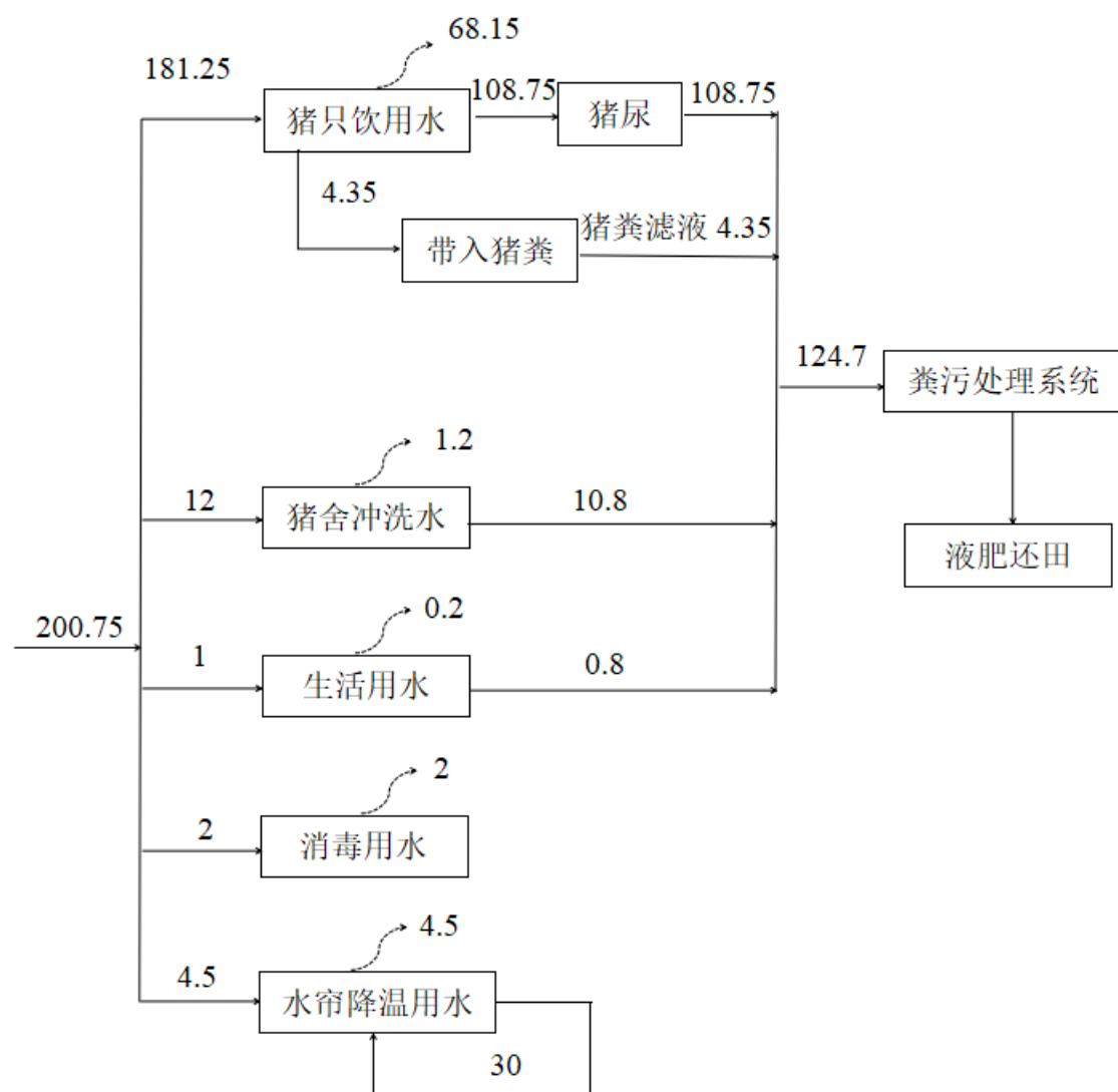
图 4.2-1 本项目水平衡图 单位: \text{m}^3/\text{d}
