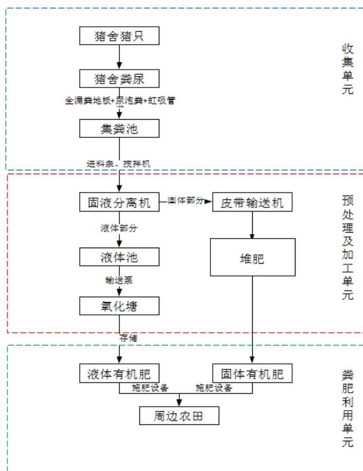
图 4.4.3 粪肥处理利用工艺流程图
