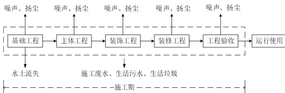
图 4.5-1 建设项目施工期工艺流程及产污环节图
