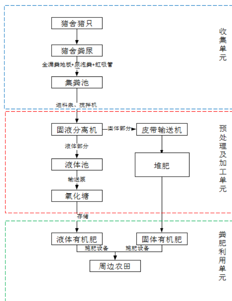
图 3.1-2 粪肥处理利用工艺流程图
