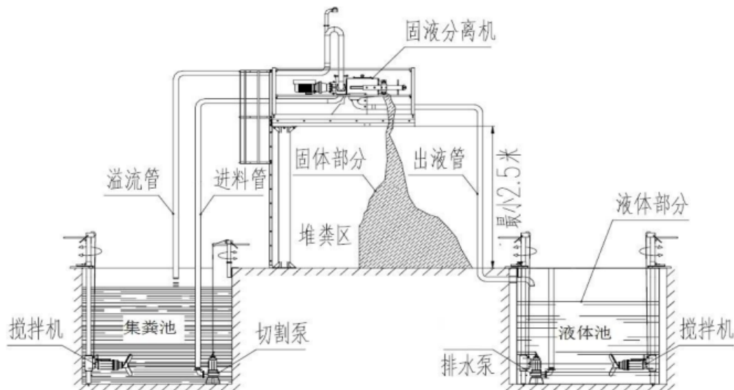
图 3.1-3 固液分离系统断面示意图
