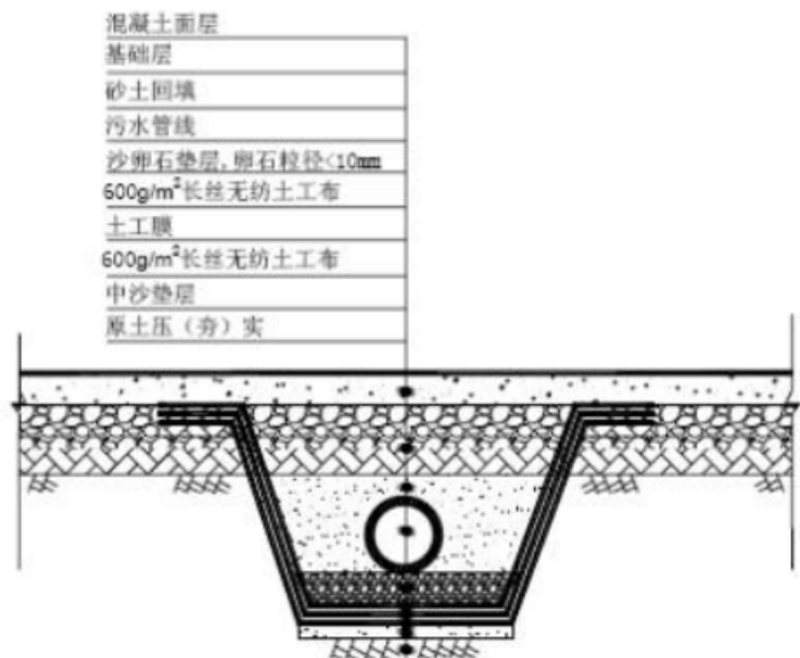
图 7.2-3 污水处理设施防渗结构
