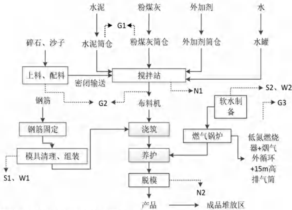
图 2-1 预制构件生产工艺流程及产污节点图
