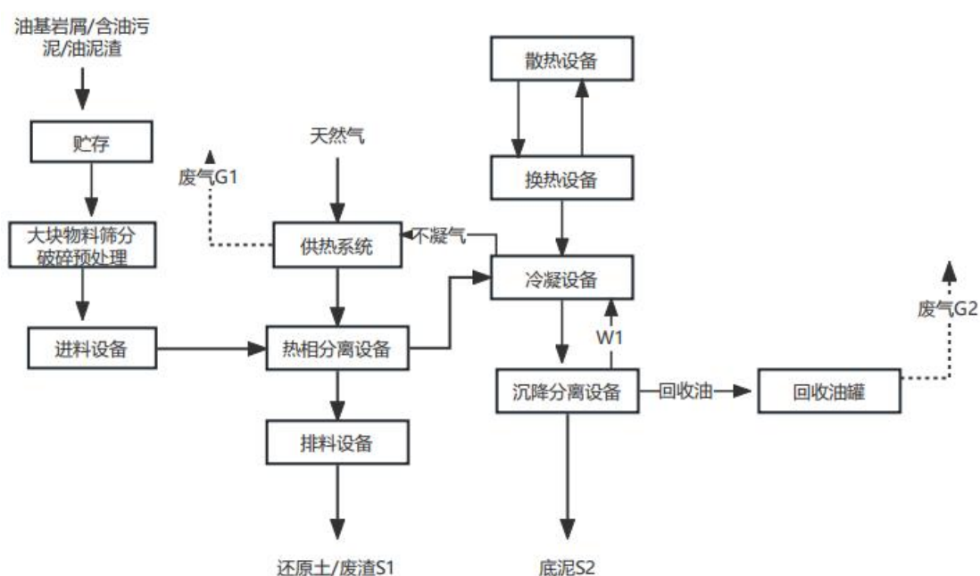
图 2-2 工艺流程图
