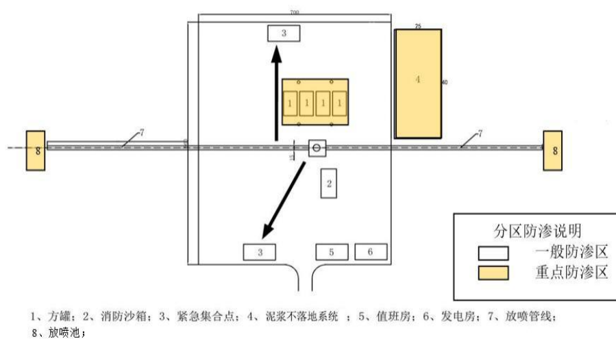
图 2-3 钻井平台井场平面布置示意图
