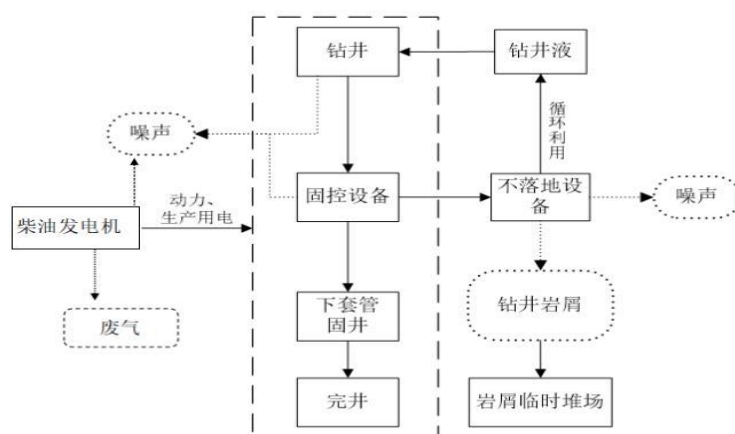
图 2-6 钻井施工作业流程及产污节点图
