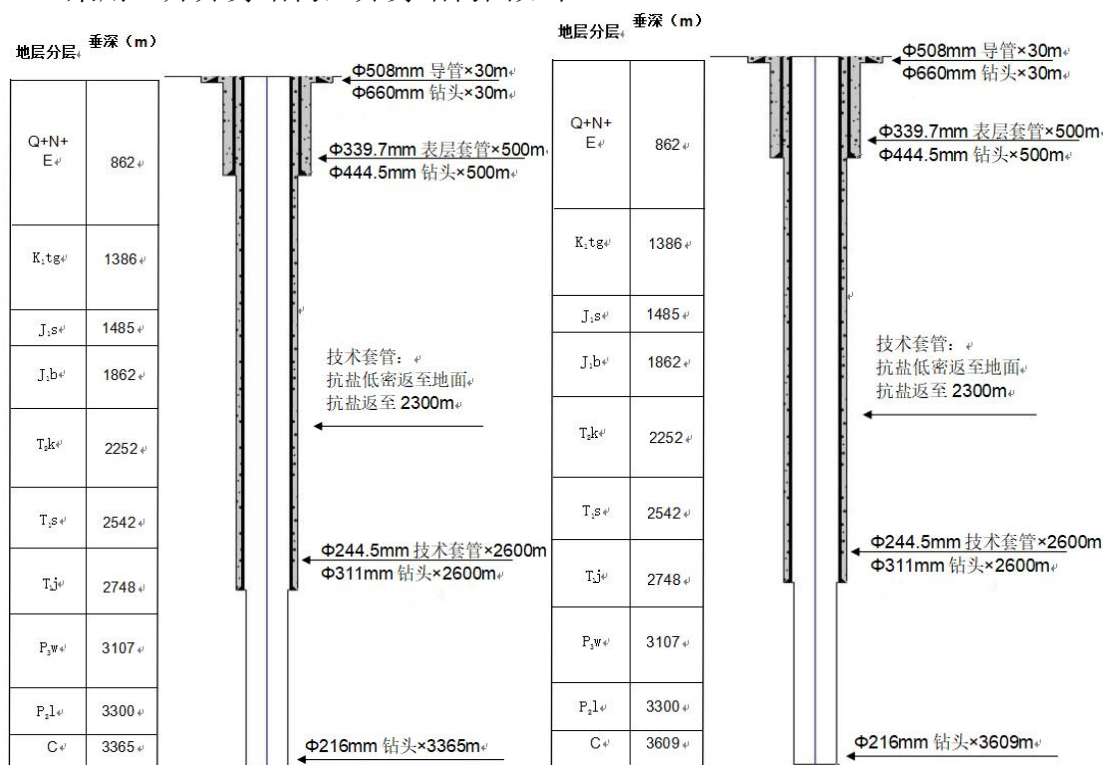
图 2-1 阜中 2 井、阜中 3 井井身结构图
