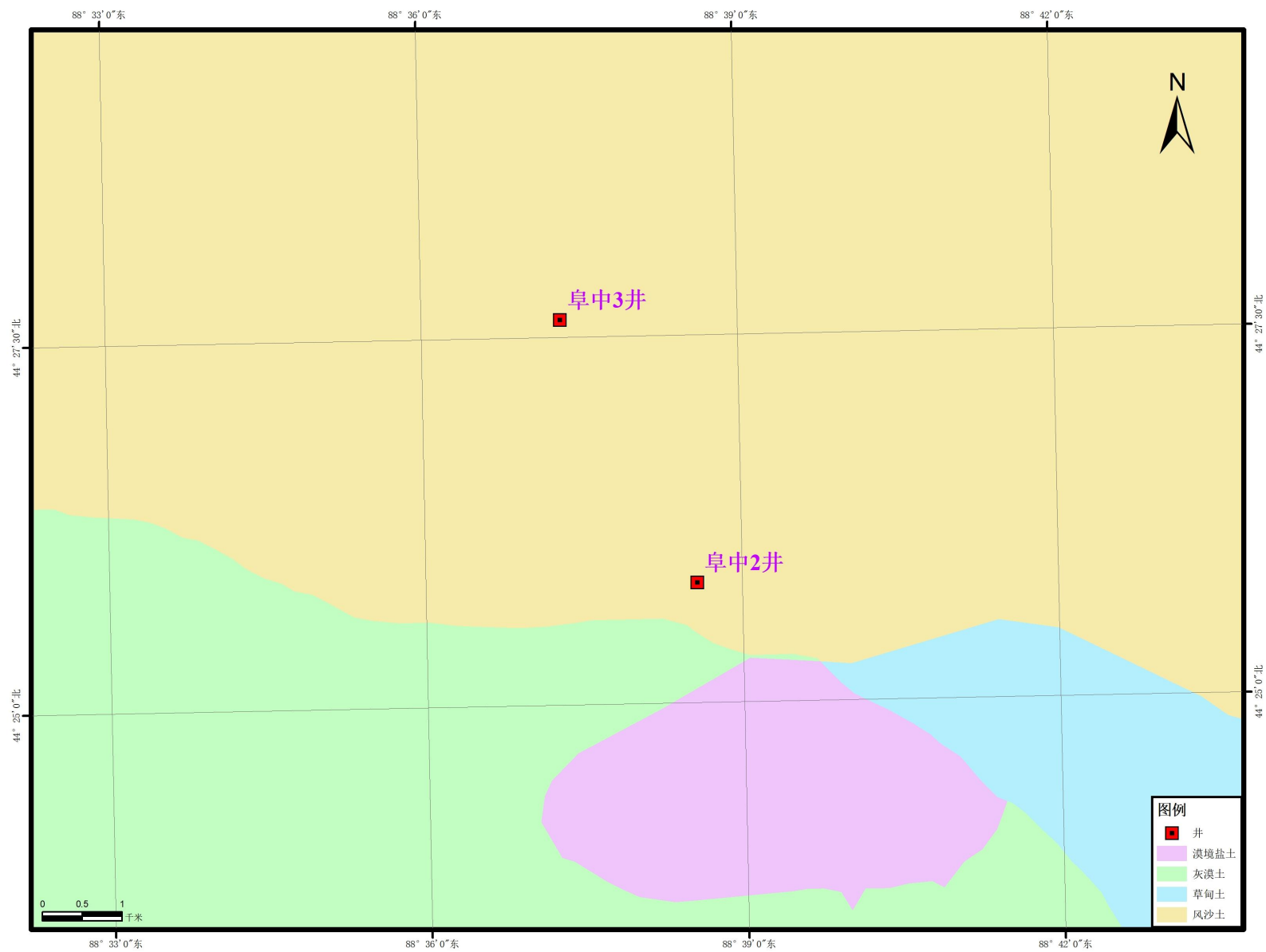
土壤类型分布图 附图 8 土壤类型图
