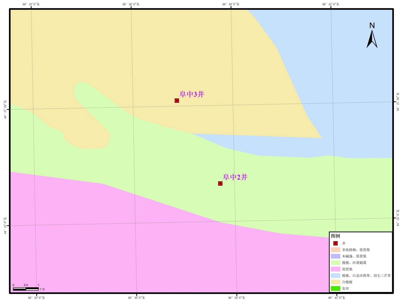
植被类型分布图
