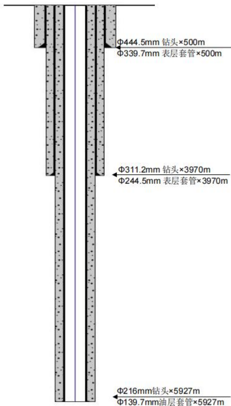
图 2-1 阜康 3 井井身结构图
