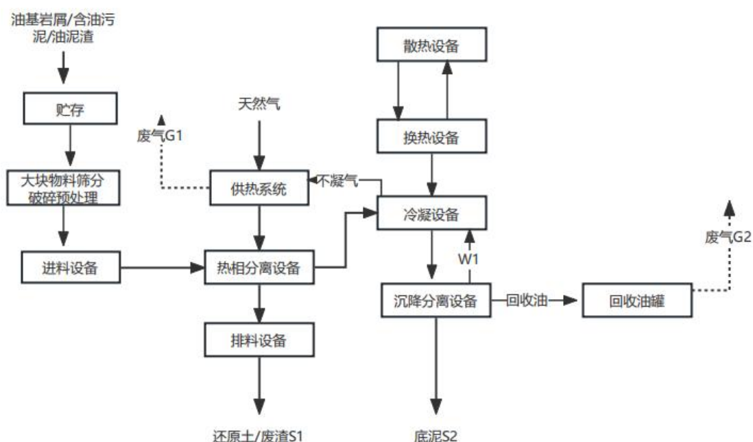
图 2-2 工艺流程图
