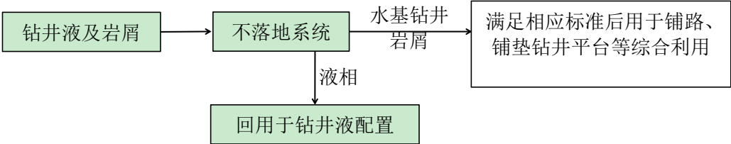
图 5-2 水基钻井岩屑处理工艺流程图
