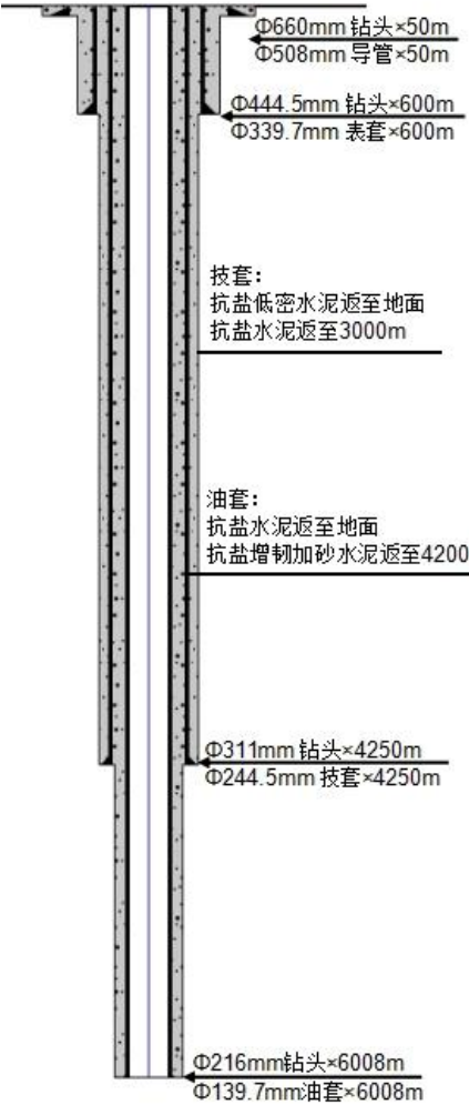
图1 井身结构示意图
