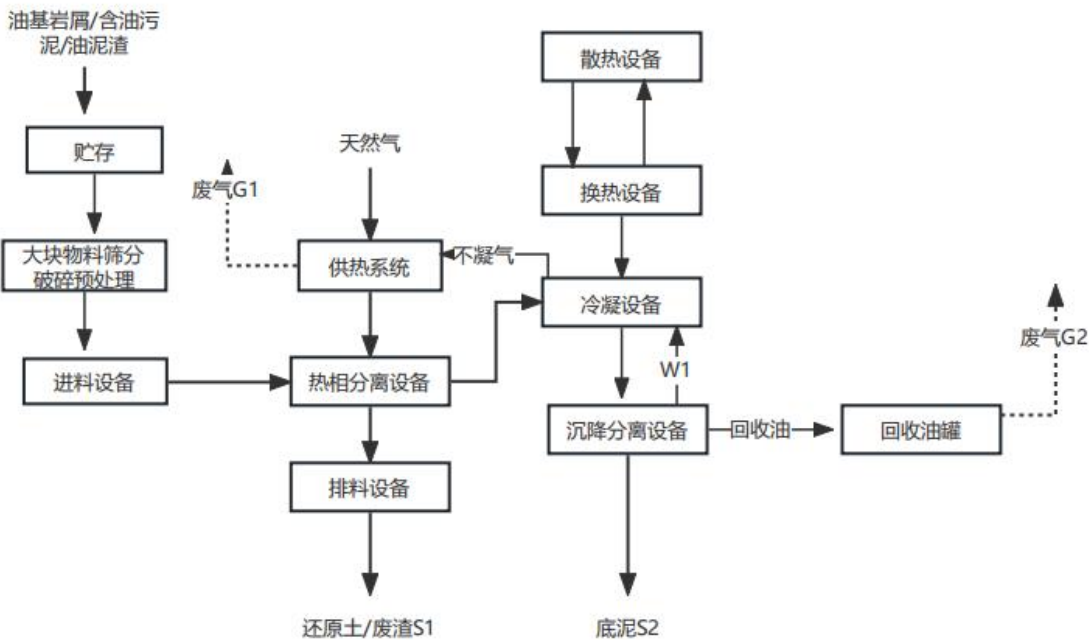
图2-6工艺流程图
