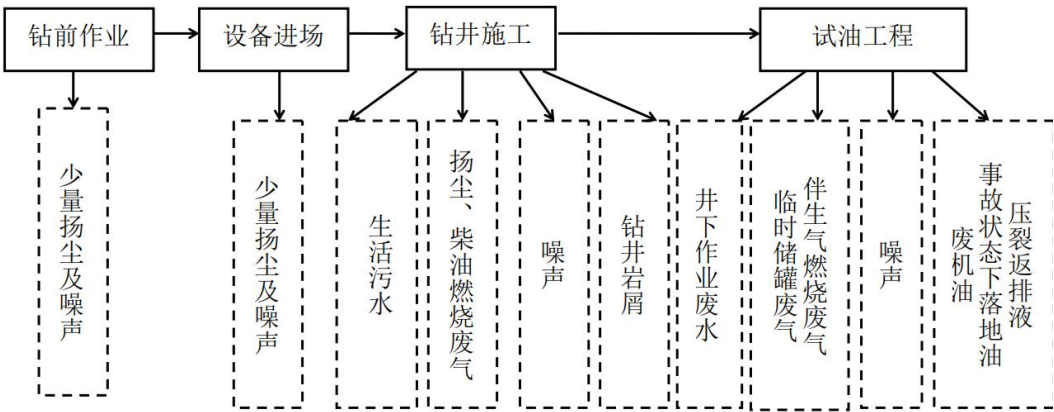
图7 钻井工艺流程及产污节点图
