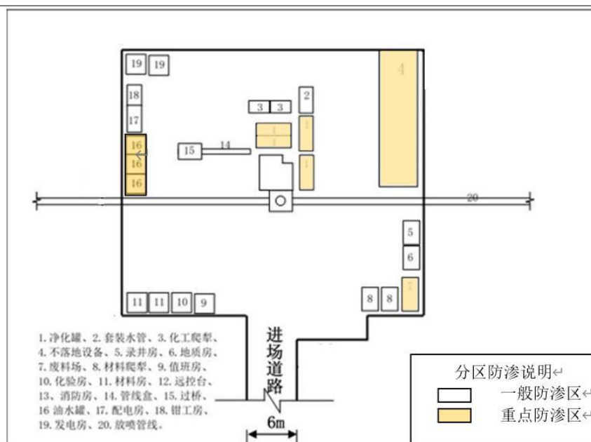
图11 分区防渗图
