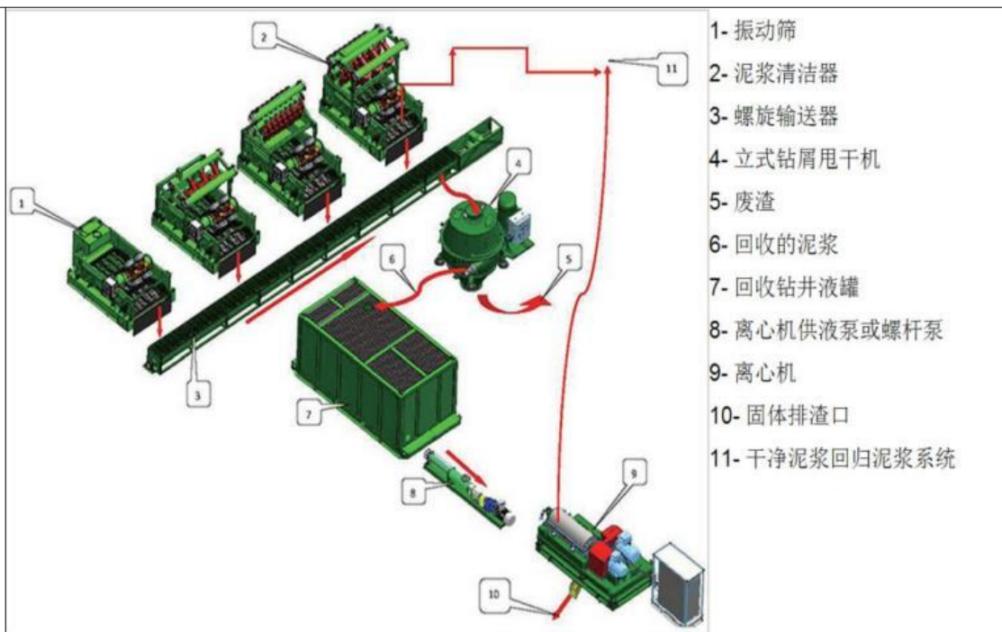
图9 钻井泥浆不落地装置示意图
