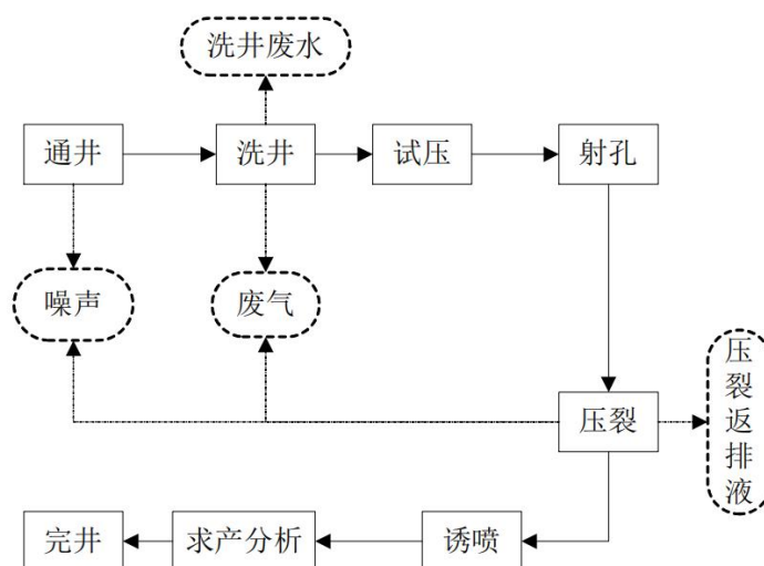
图10 试油作业流程及产污节点图
