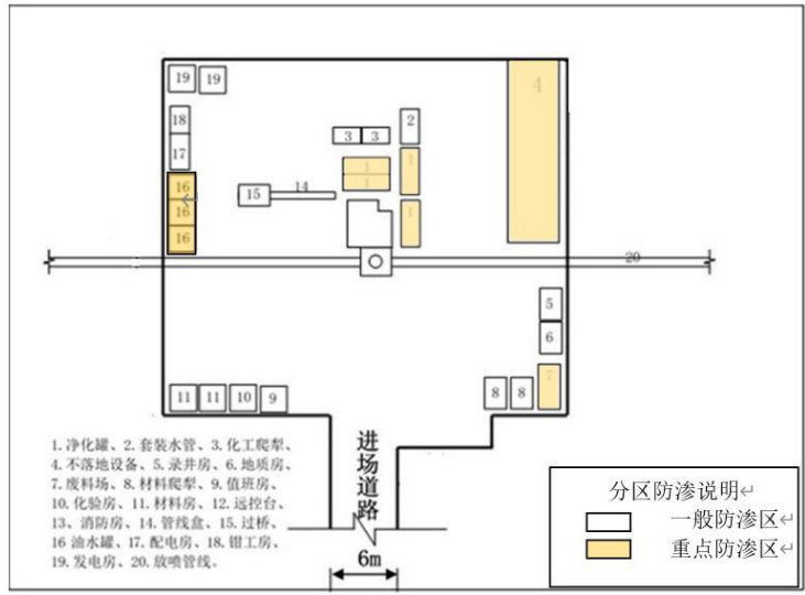
图6 油气测试井场平面布置图示意图
