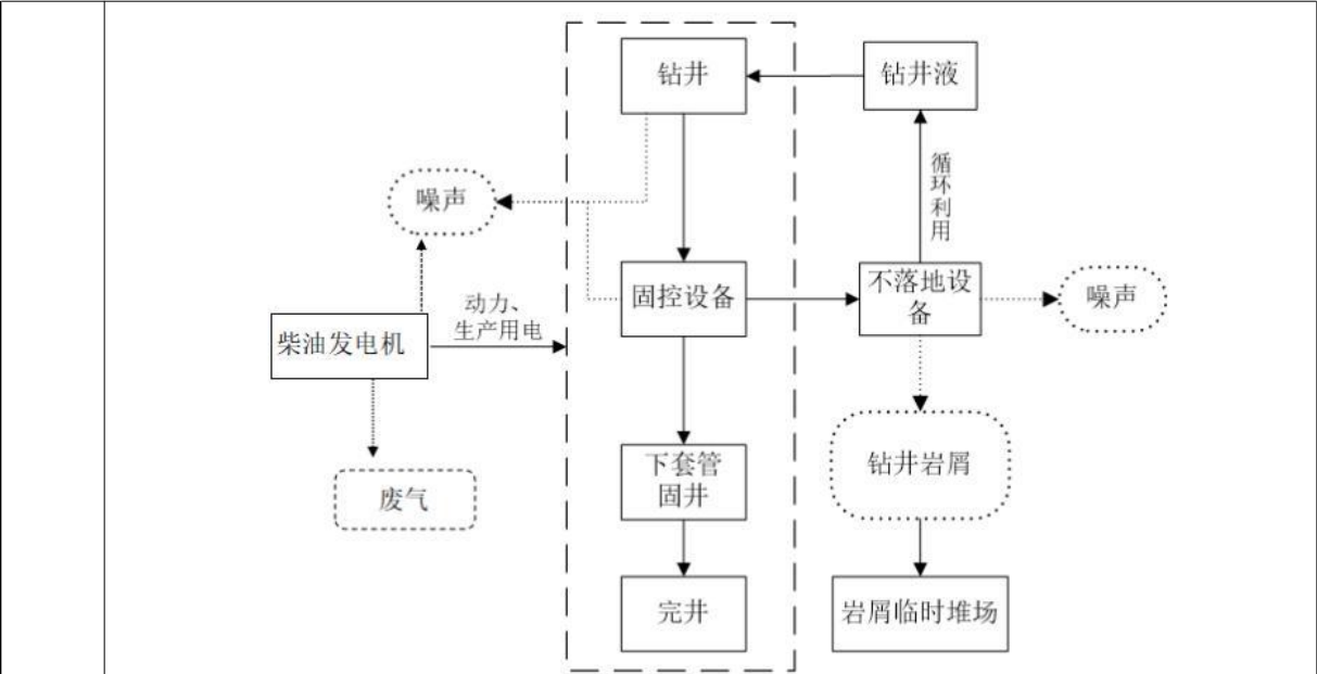
图8 钻井施工作业流程及产污节点图
