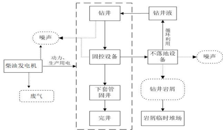
图 2-6 钻井施工作业流程及排污节点图
