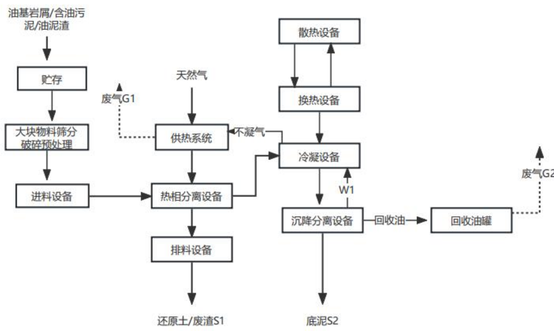
图 2-2 工艺流程图
