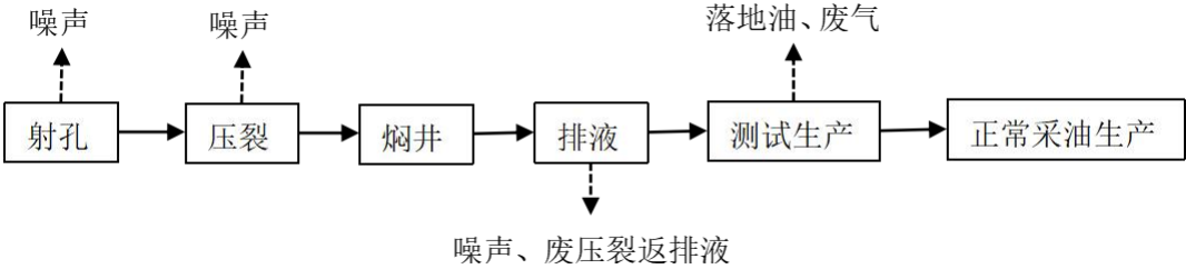
图 2-8 压裂作业工艺流程及产污环节图
