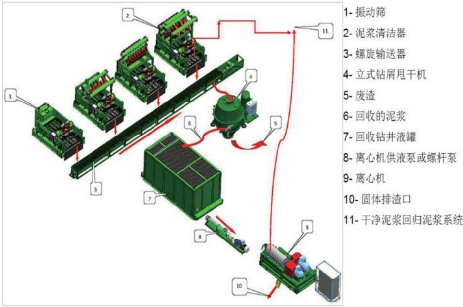
图 2-7 钻井泥浆不落地装置示意图
