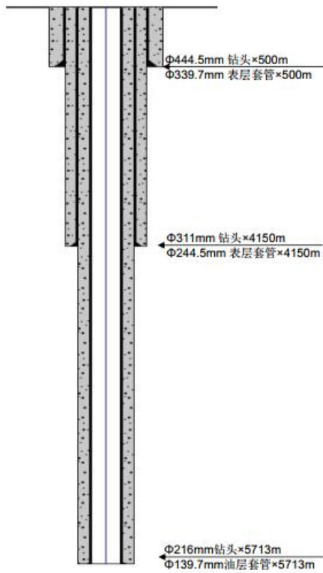
图 2-1 阜 5301H 井井身结构图
