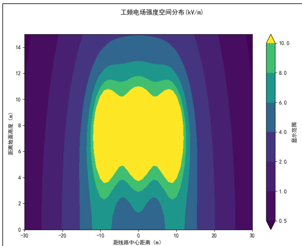
图 15 220kV 单回架空线路居民区工频电场强度等值线图
