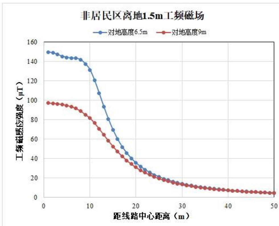
图 20 220kV 单回架空线路抬升至 9m 后工频磁感应强度预测结果图
