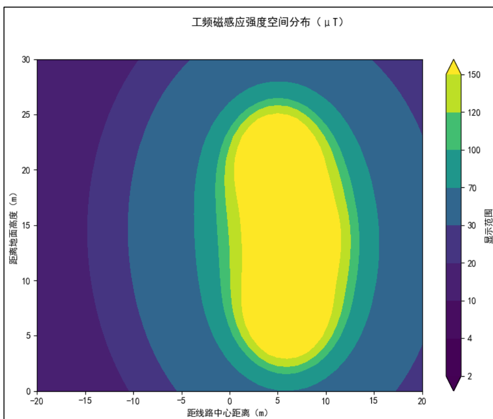
图 29 220kV 双回线路（本期单边挂线）非居民区工频磁感应强度等值线图
