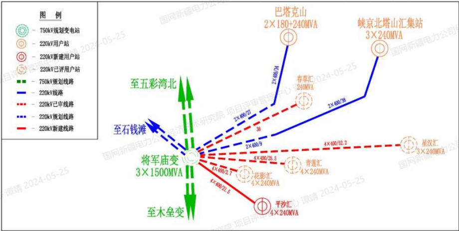
昌吉平沙升压汇集站220千伏送出工程电网接线示意图
