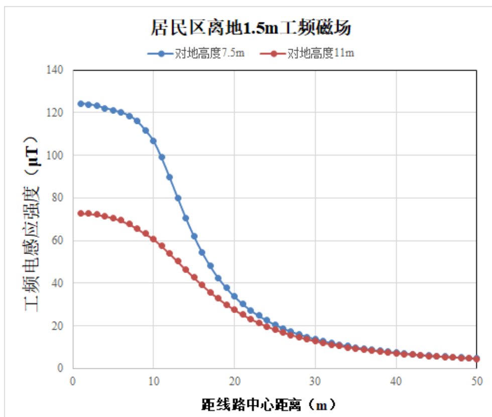
图 24 220kV 单回架空线路抬升至 11m 后工频磁感应强度预测结果图
