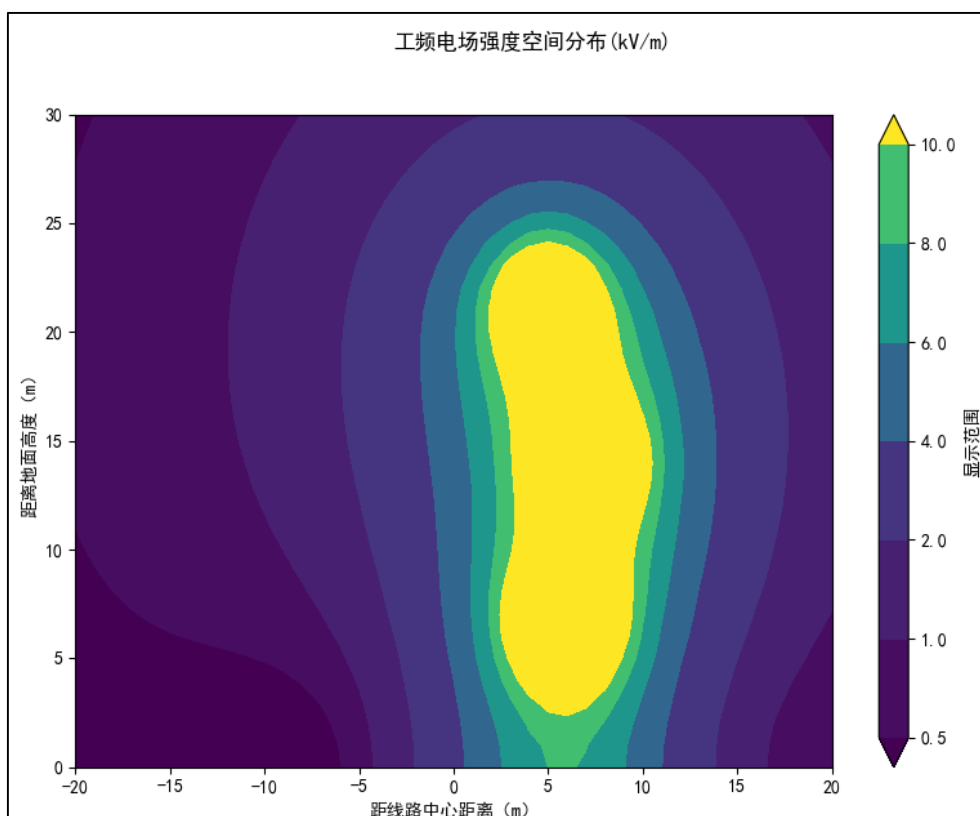
图 27 220kV 双回线路（本期单边挂线）非居民区工频电场强度等值线图
