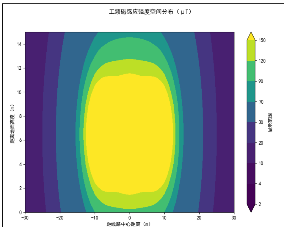
图 13 220kV 单回架空线路非居民区工频磁感应强度等值线图
