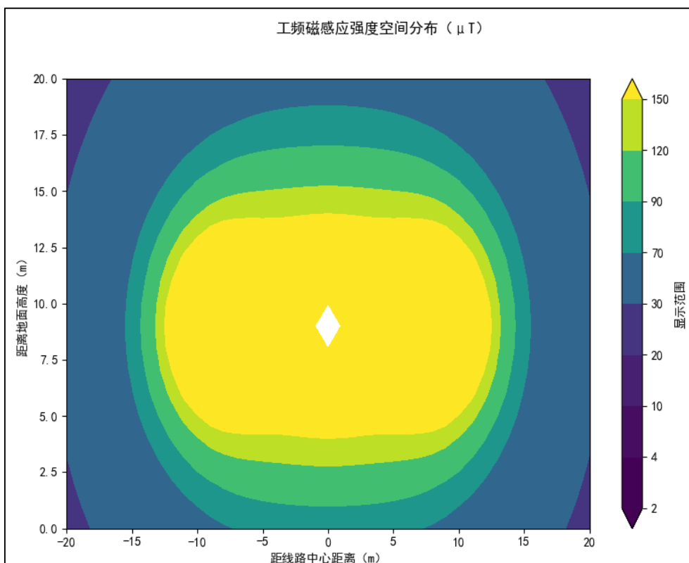
图 21 220kV 单回架空线路抬升至 9m 后工频磁感应强度等值线图
