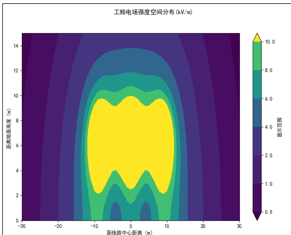
图 11 220kV 单回架空线路非居民区工频电场强度等值线图
