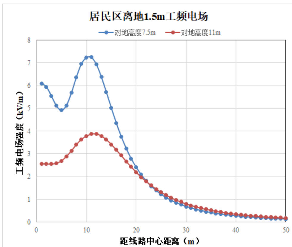
图 22 220kV 单回架空线路抬升至 11m 后工频电场强度预测结果图
