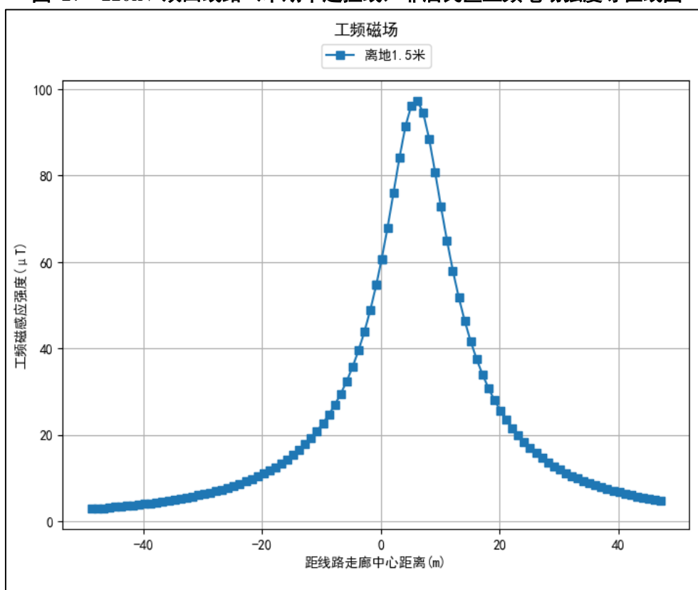
图 28 220kV 双回线路（本期单边挂线）非居民区工频磁感应强度预测结果图
