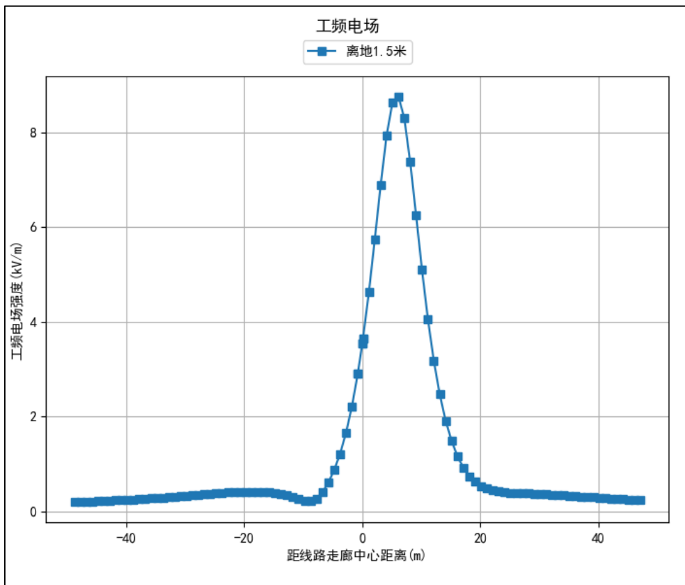
图 26 220kV 双回线路（本期单边挂线）非居民区工频电场强度预测结果图
