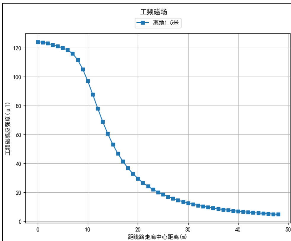
图 16 220kV 单回架空线路居民区工频磁感应强度预测结果图
