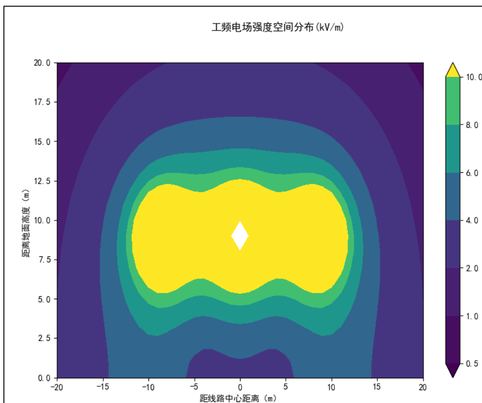
图 19 220kV 单回架空线路抬升至 9m 后工频电场强度等值线图
