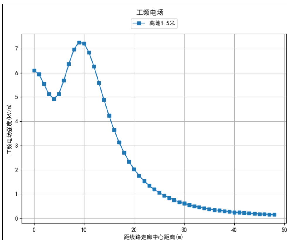
图 14 220kV 单回架空线路居民区工频电场强度预测结果图
