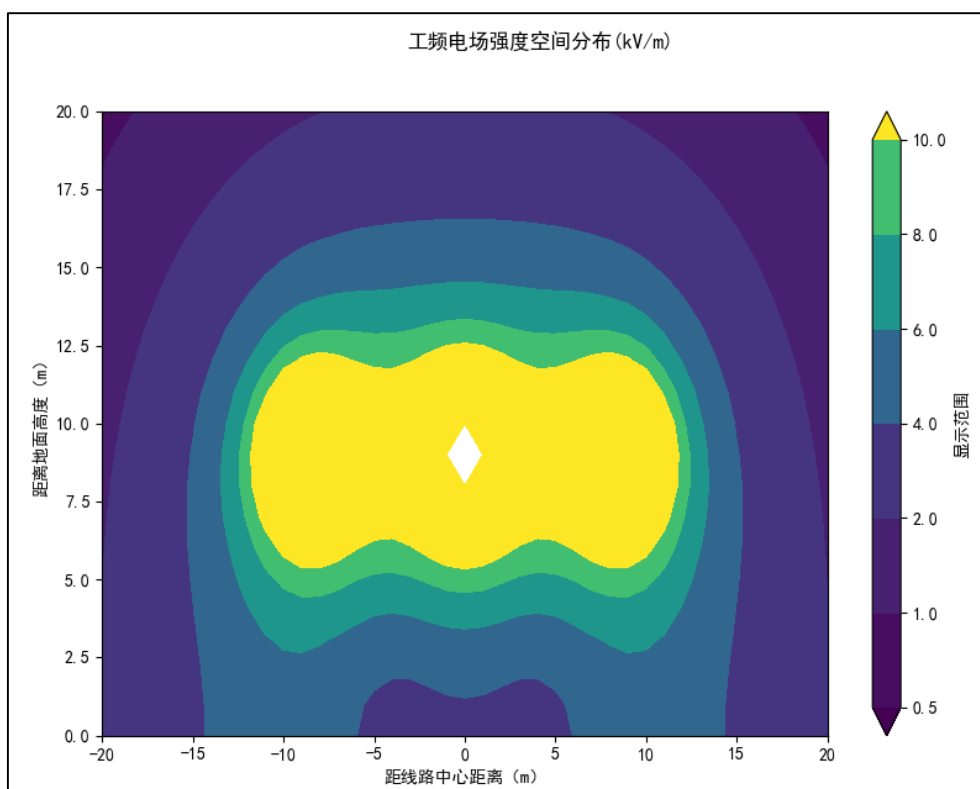
图 23 220kV 单回架空线路抬升至 11m 后工频电场强度等值线图
