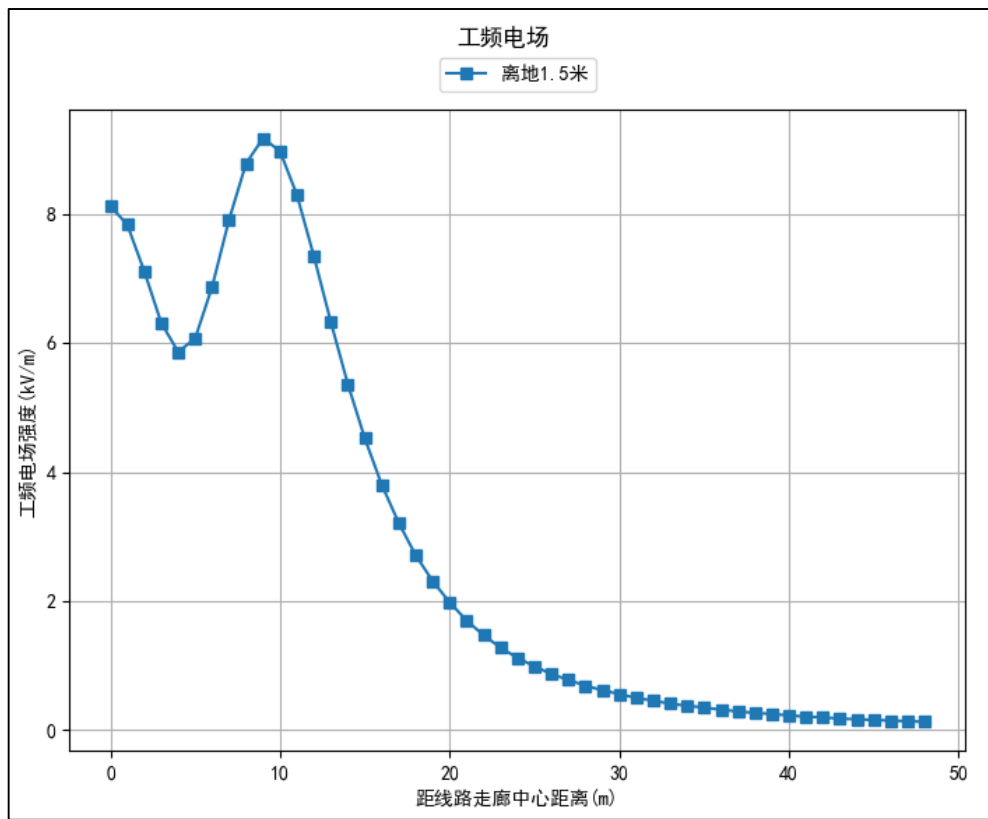
图 10 220kV 单回架空线路非居民区工频电场强度预测结果图
