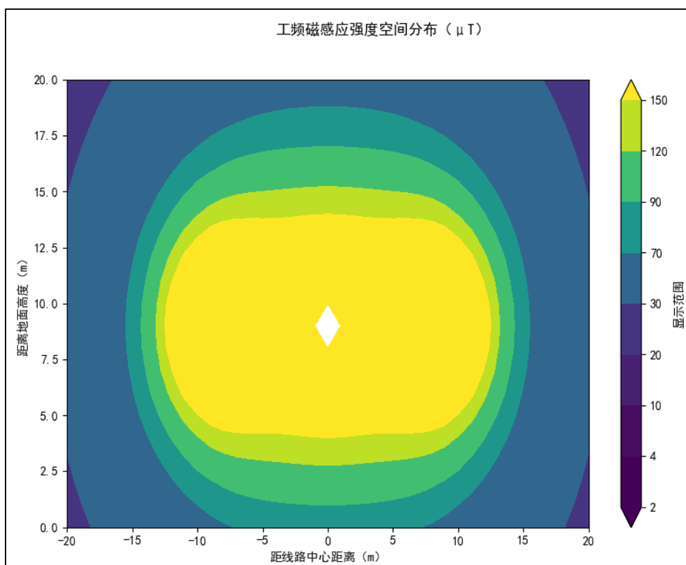
图 25 220kV 单回架空线路抬升至 11m 后工频磁感应强度等值线图
