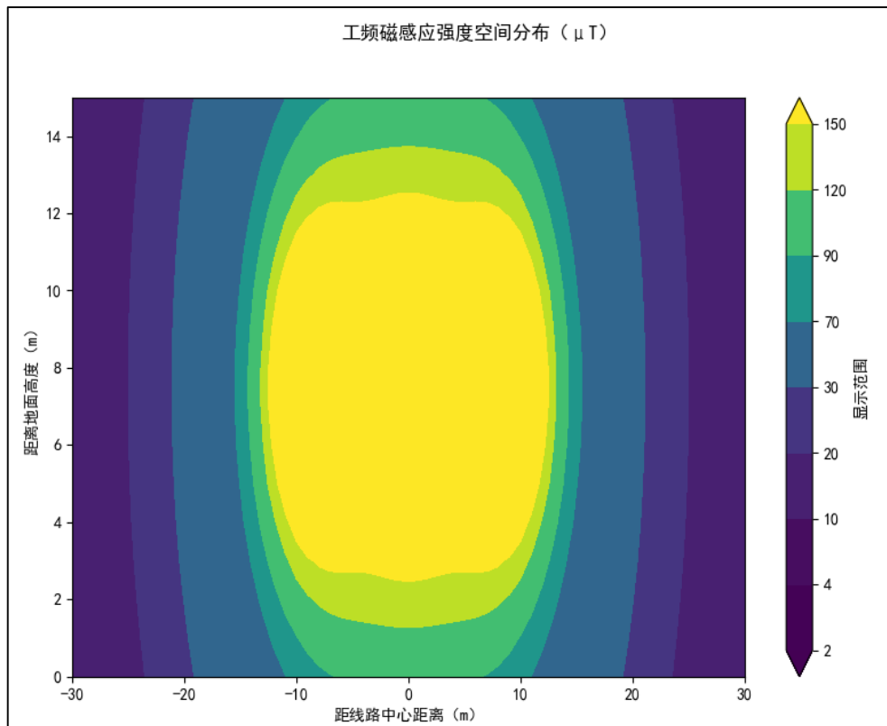
图 17 220kV 单回架空线路居民区工频磁感应强度等值线图
