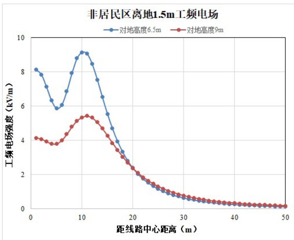
图 18 220kV 单回架空线路抬升至 9m 后的工频电场强度预测结果图
