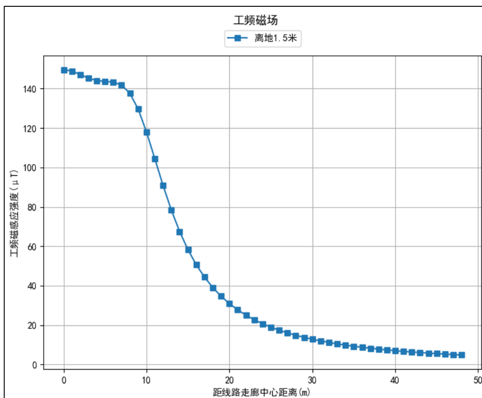
图 12 220kV 单回架空线路非居民区工频磁感应强度预测结果图
