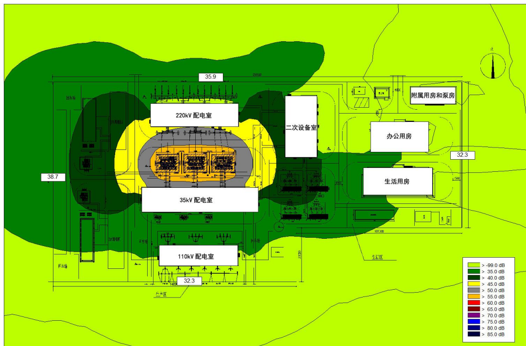
图 9 升压站噪声预测图
