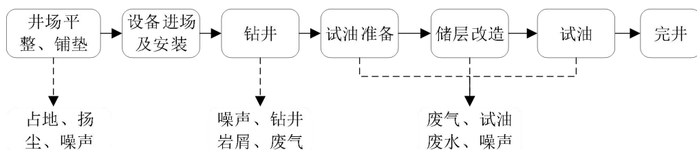
图 1 工艺流程及产污环节示意图
