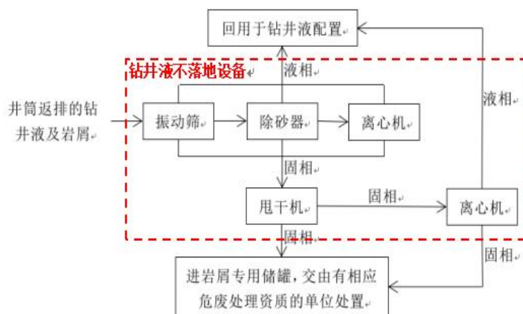
图3 油基钻井岩屑不落地系统工艺流程示意图
