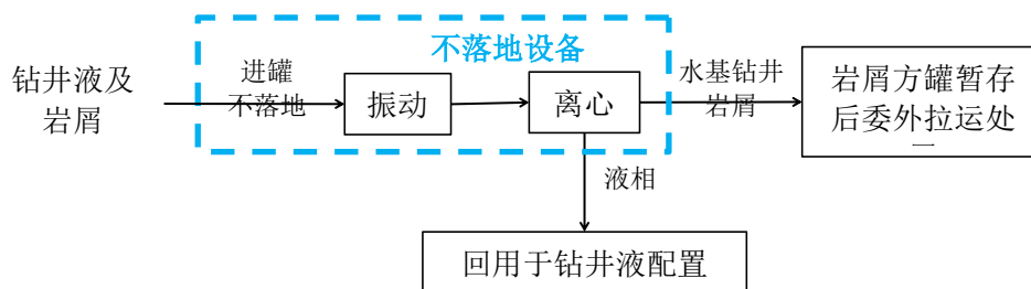
图2 水基钻井岩屑井场处理工艺流程
