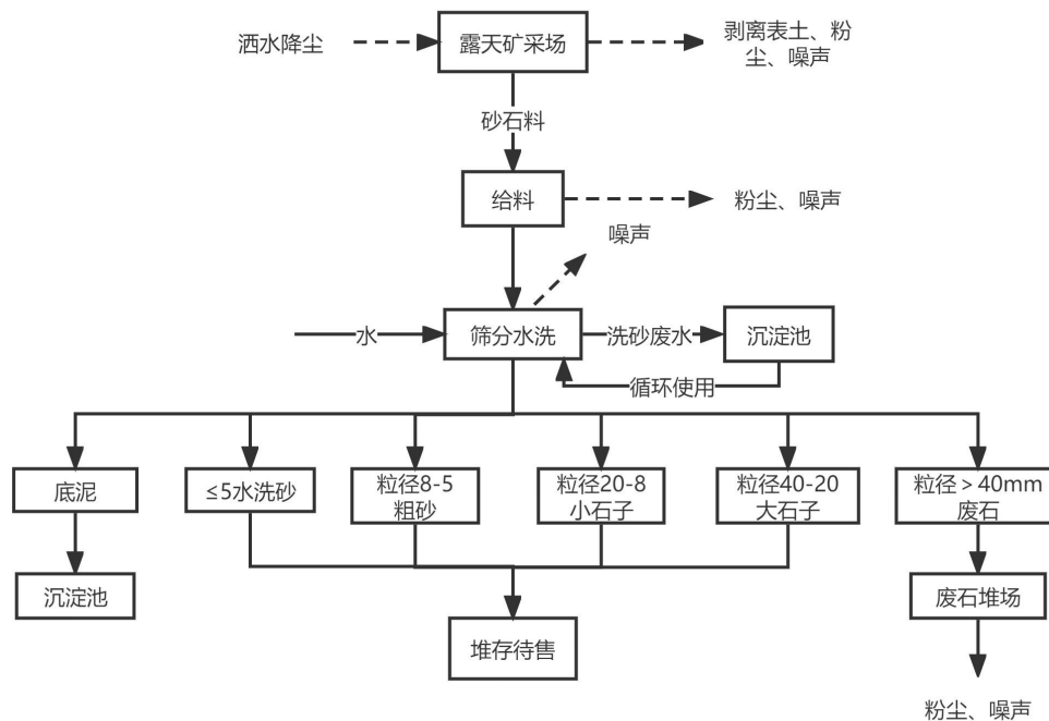
图3 项目生产工艺及产污环节示意图
