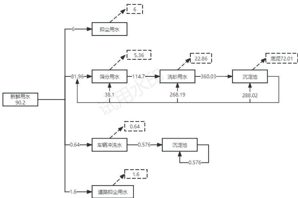
图 1 本项目水平衡图 单位：m³/d
