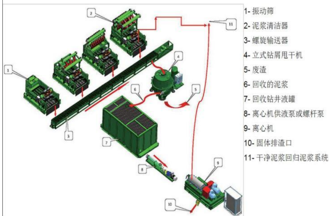
图8 钻井泥浆不落地装置示意图
