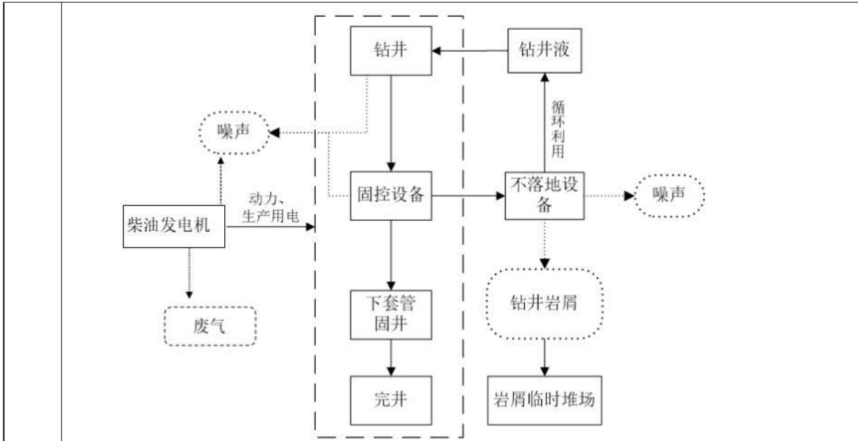
图7 钻井施工作业流程及产污节点图
