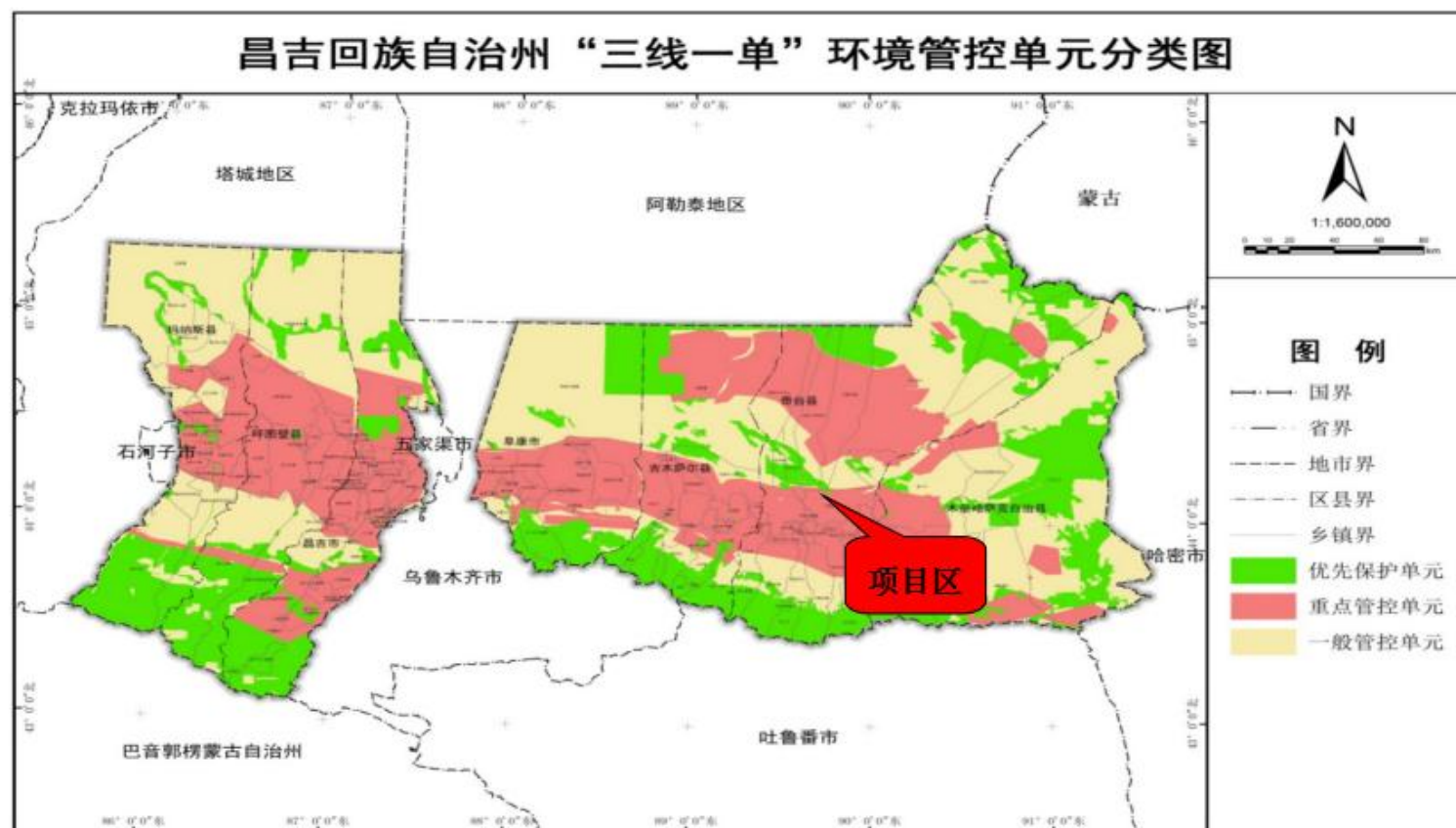
附图 2 昌吉州环境管控单元分类
