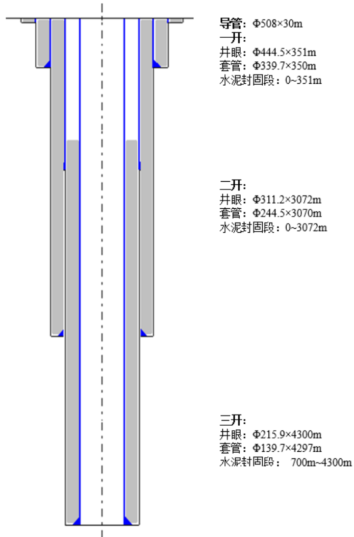
图 1 钻井井身结构图
