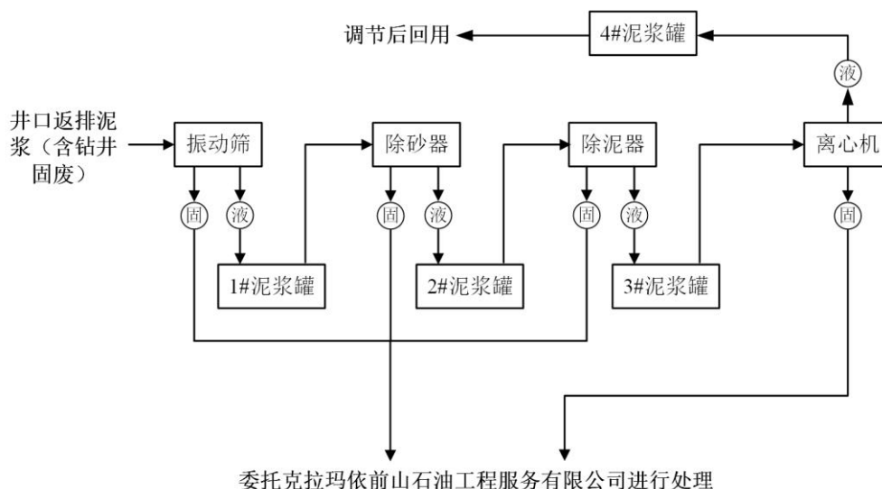
图 5 “泥浆不落地”工艺原理示意图
