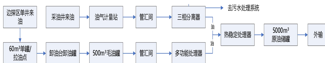
图 3 沙南联合站原油处理系统工艺流程示意图
