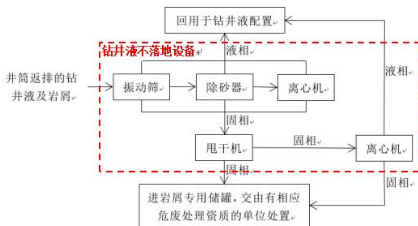
图 5 油基钻井岩屑不落地系统工艺流程示意图
