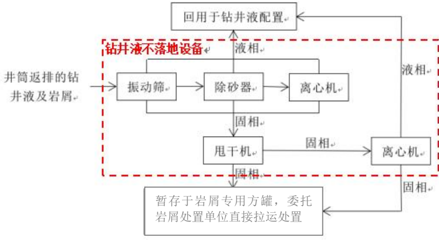
图 4 水基钻井岩屑处理工艺流程图
