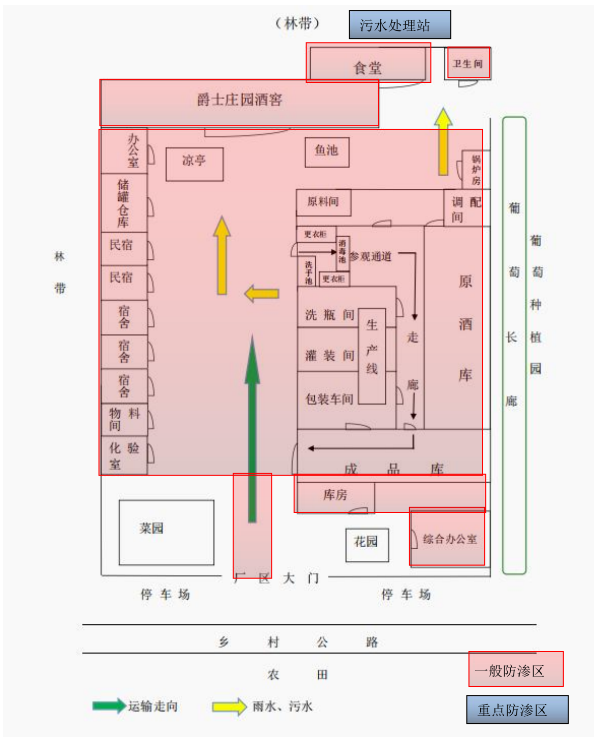
图 4-1 分区防渗图
