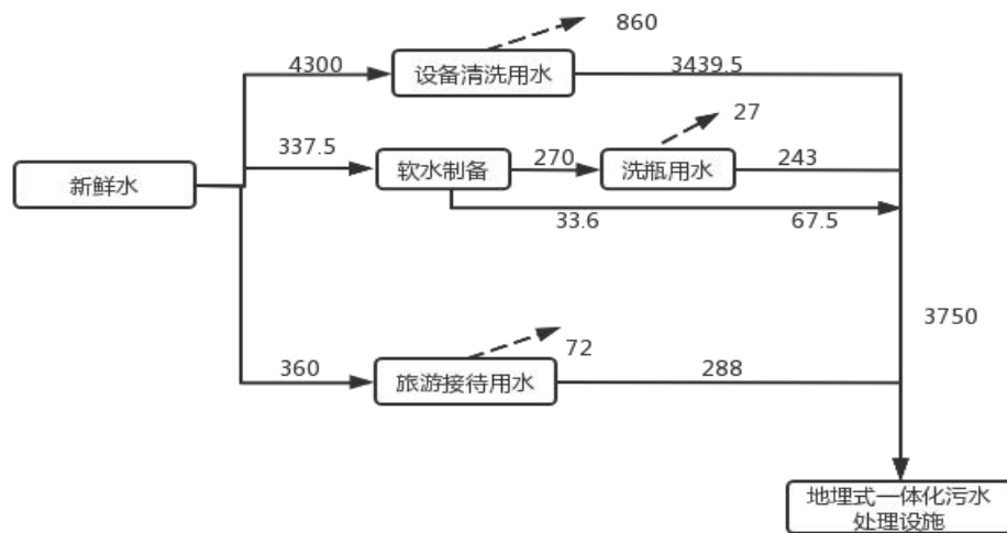
附图 2-3 水平衡图 单位 t/a
