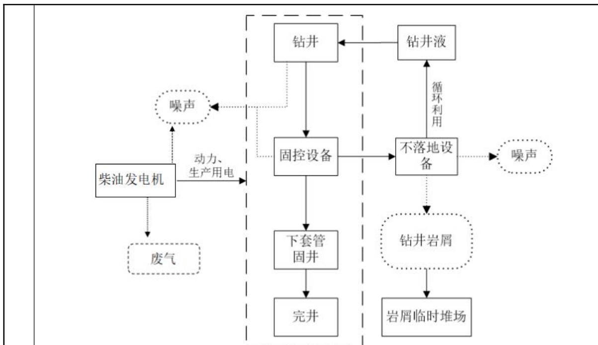
图 2-6 钻井施工作业流程及产污节点图
