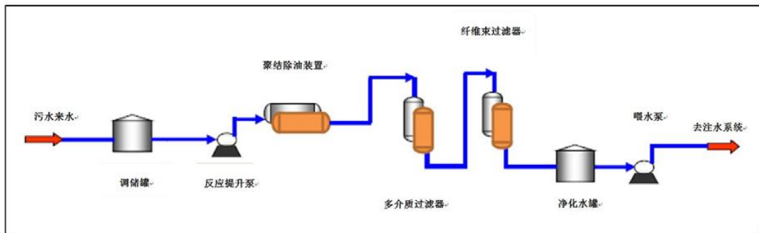
图 2-2 污水处理工艺流程图
