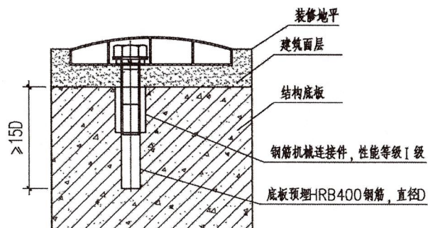
弧形门槛底部连接做法示意
