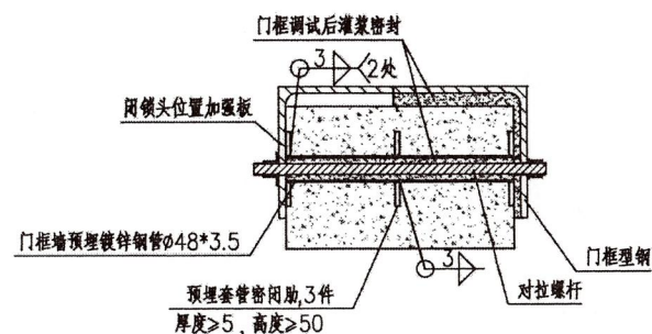
门框闭锁加强连接做法示意图
