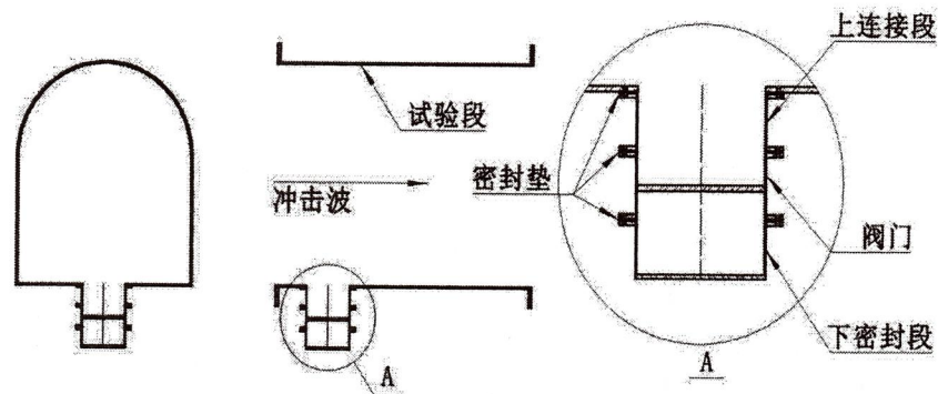
图 B. 4 阀门固定方式示意图
