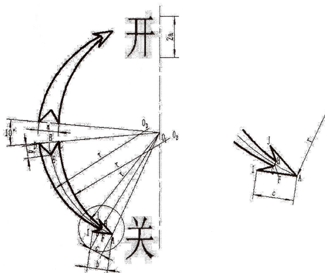
图5 开关指示箭形标志尺寸示例
