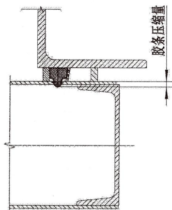
图1 挤压式
