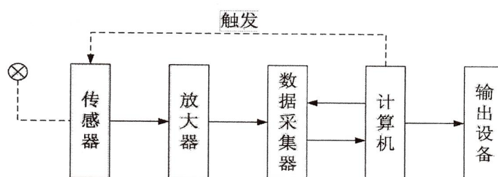
图 A. 1 测试系统工作原理示意图
