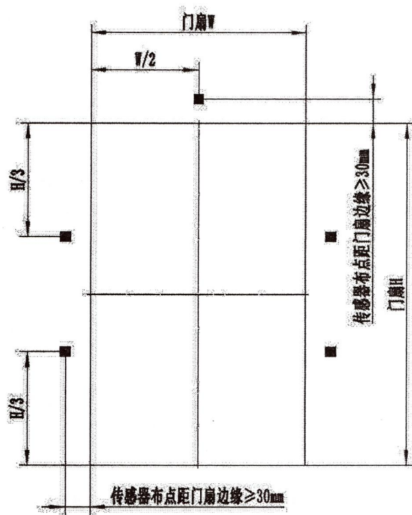
图A.4 传感器布点示意图
