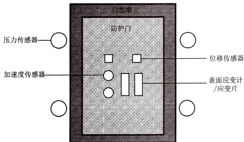
(b) 传感器布置图
