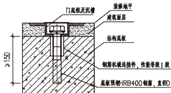
无门槛底部连接做法示意
