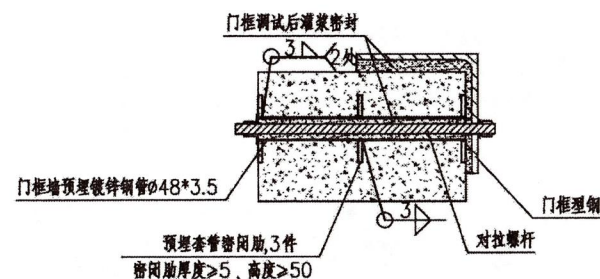
门框连接做法示意图
