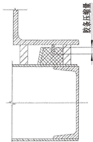
图2 嵌压式
