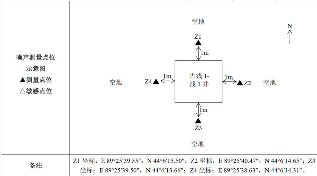
图 3 声环境监测布点示意图
