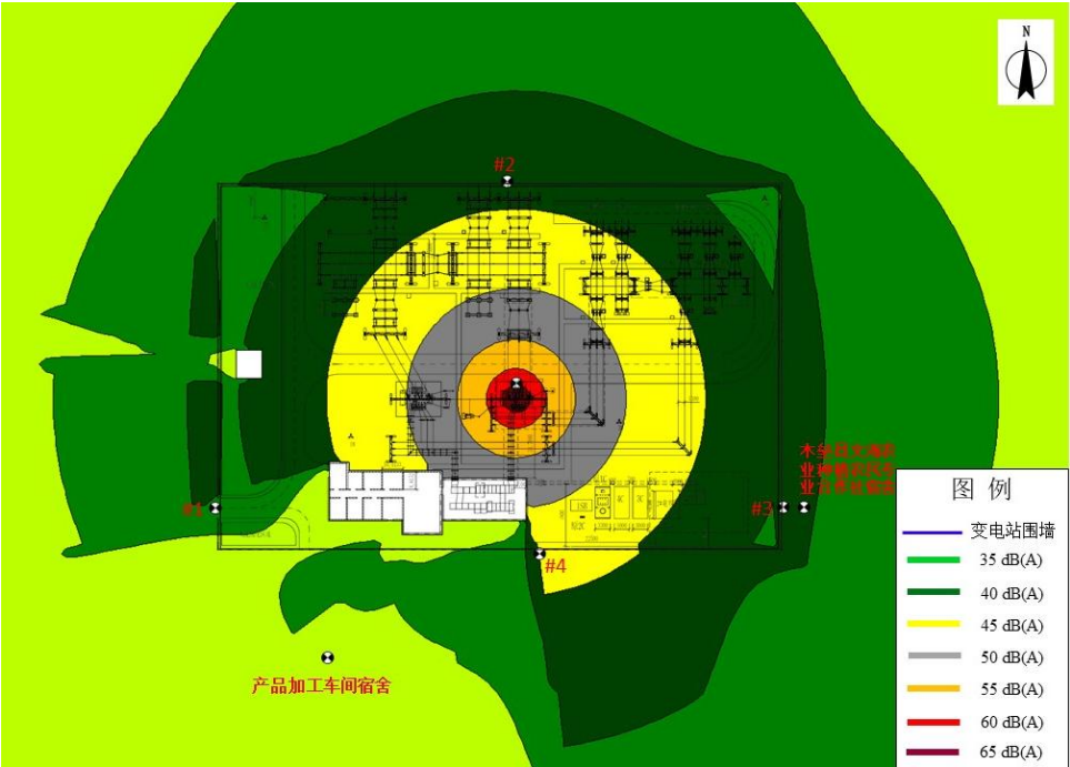
图 6 变电站本期改建规模噪声预测的声等值线图
