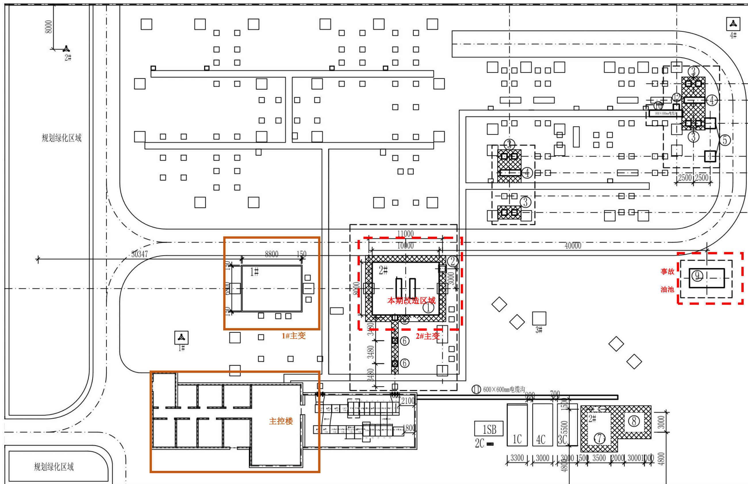
附图 2: 昌吉木垒 110kV 变电站总平面布置示意图
