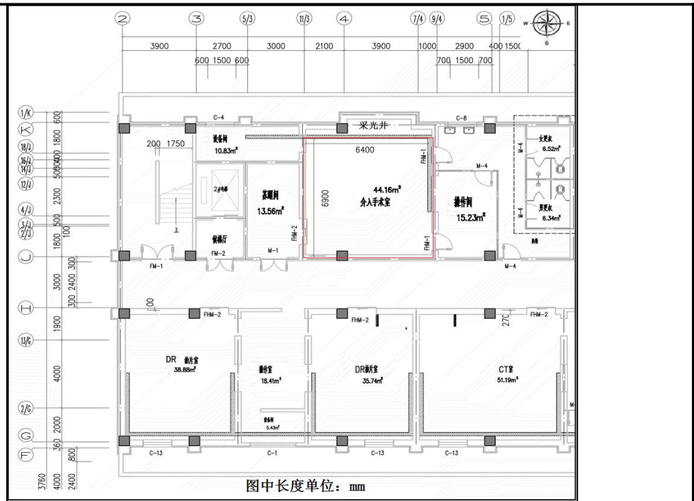
图1-3 拟建 DSA机房平面布置示意图
