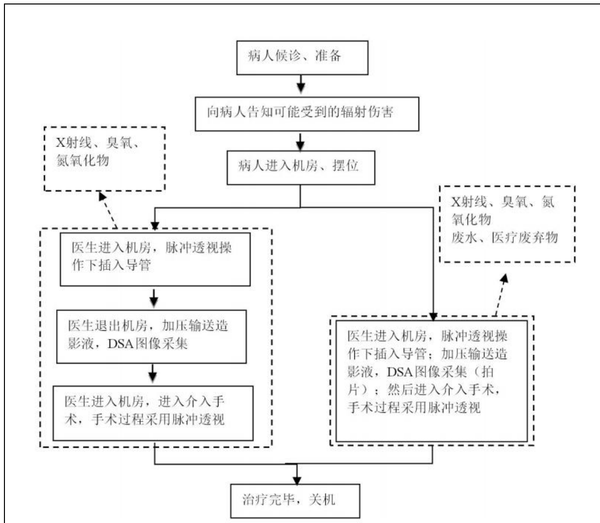
图9-2 DSA工艺流程及产污环节图
