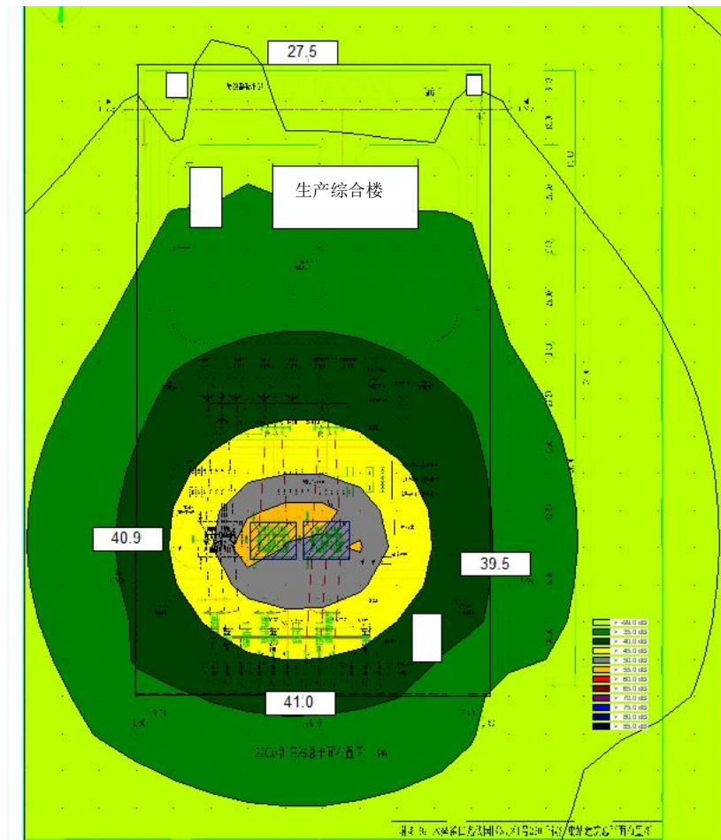
图 4-1 汇集站噪声预测图
