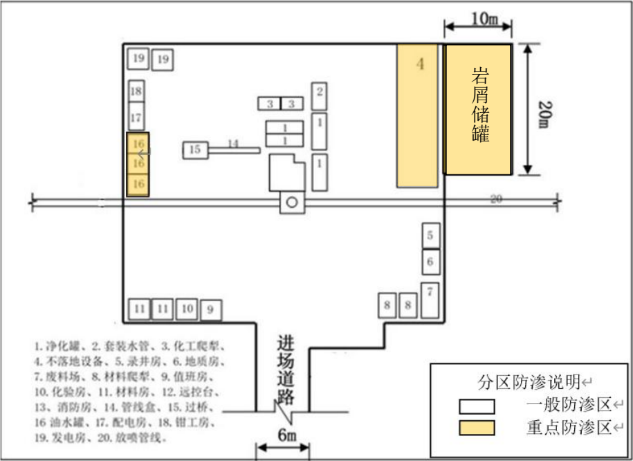
图 2-11 钻井井场平面布置示意图
