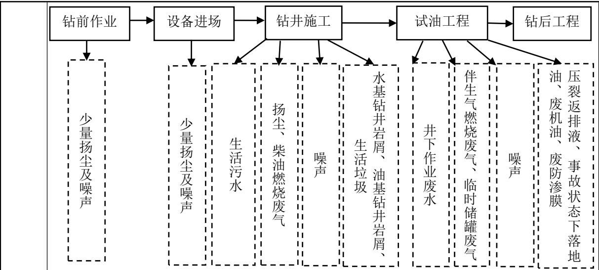
图 2-13 钻井工艺流程及产污节点图
