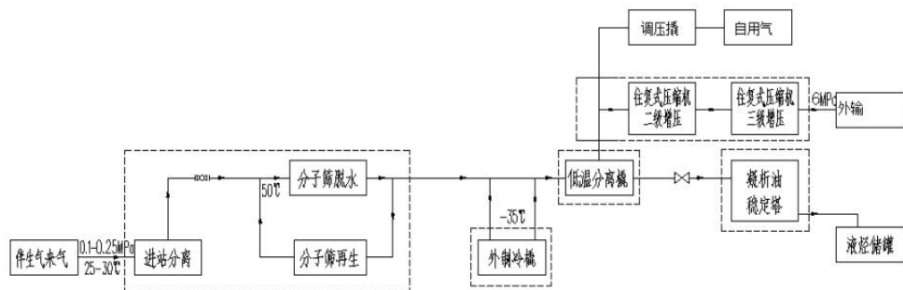
图 2-8 天然气处理系统工艺流程示意图
