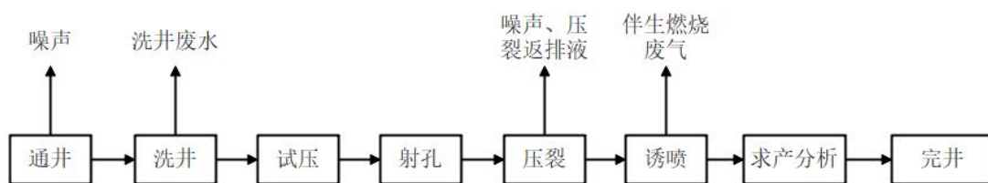
图 2-16 试油作业流程及产污节点图
