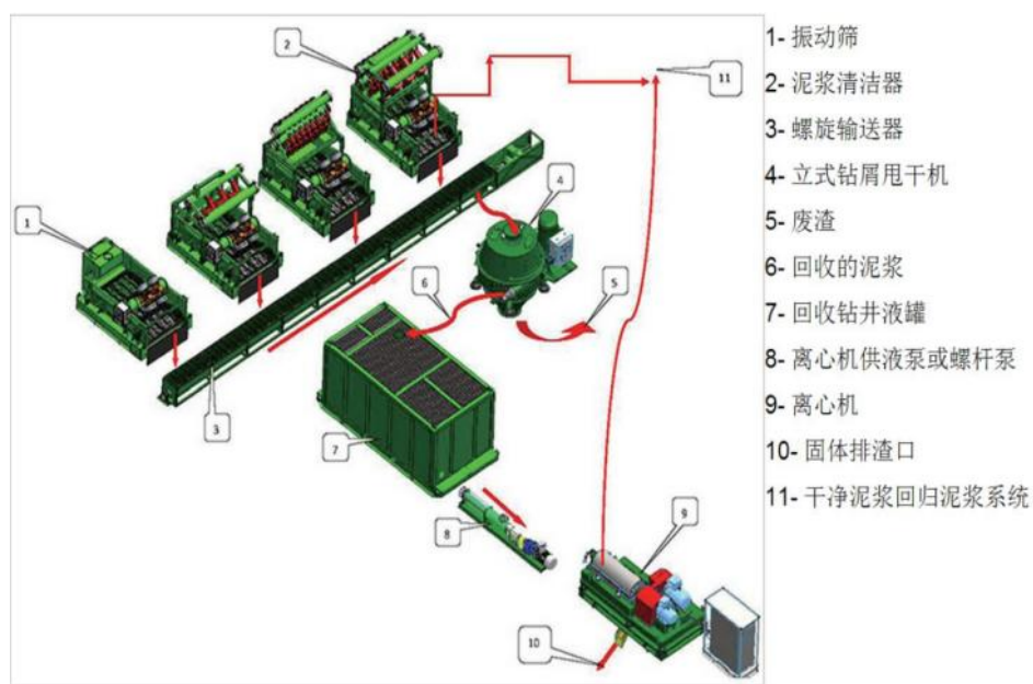
图 2-15 泥浆不落地处理系统工艺流程
