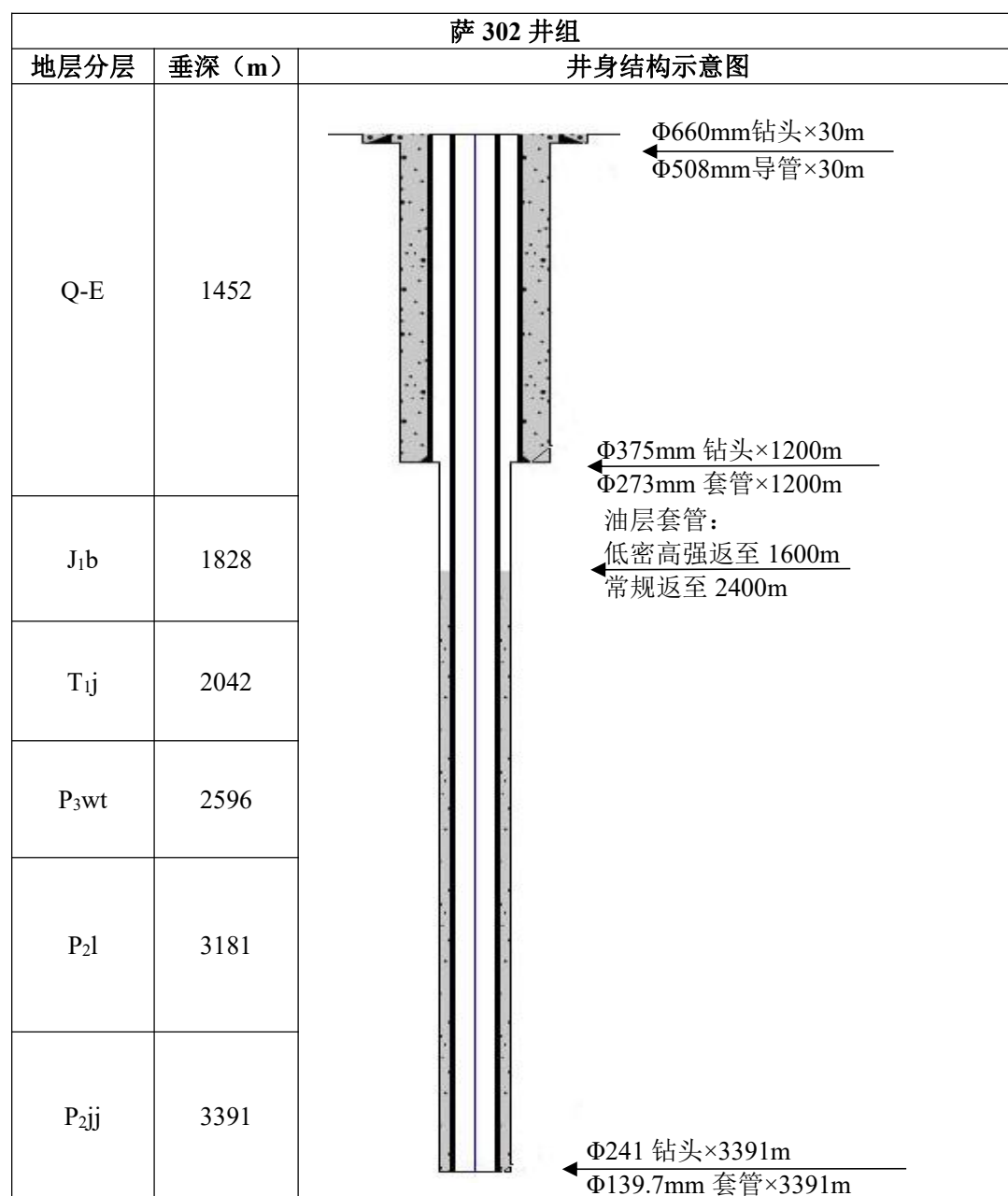
图 2-5 萨 302 井组直井井身结构图
