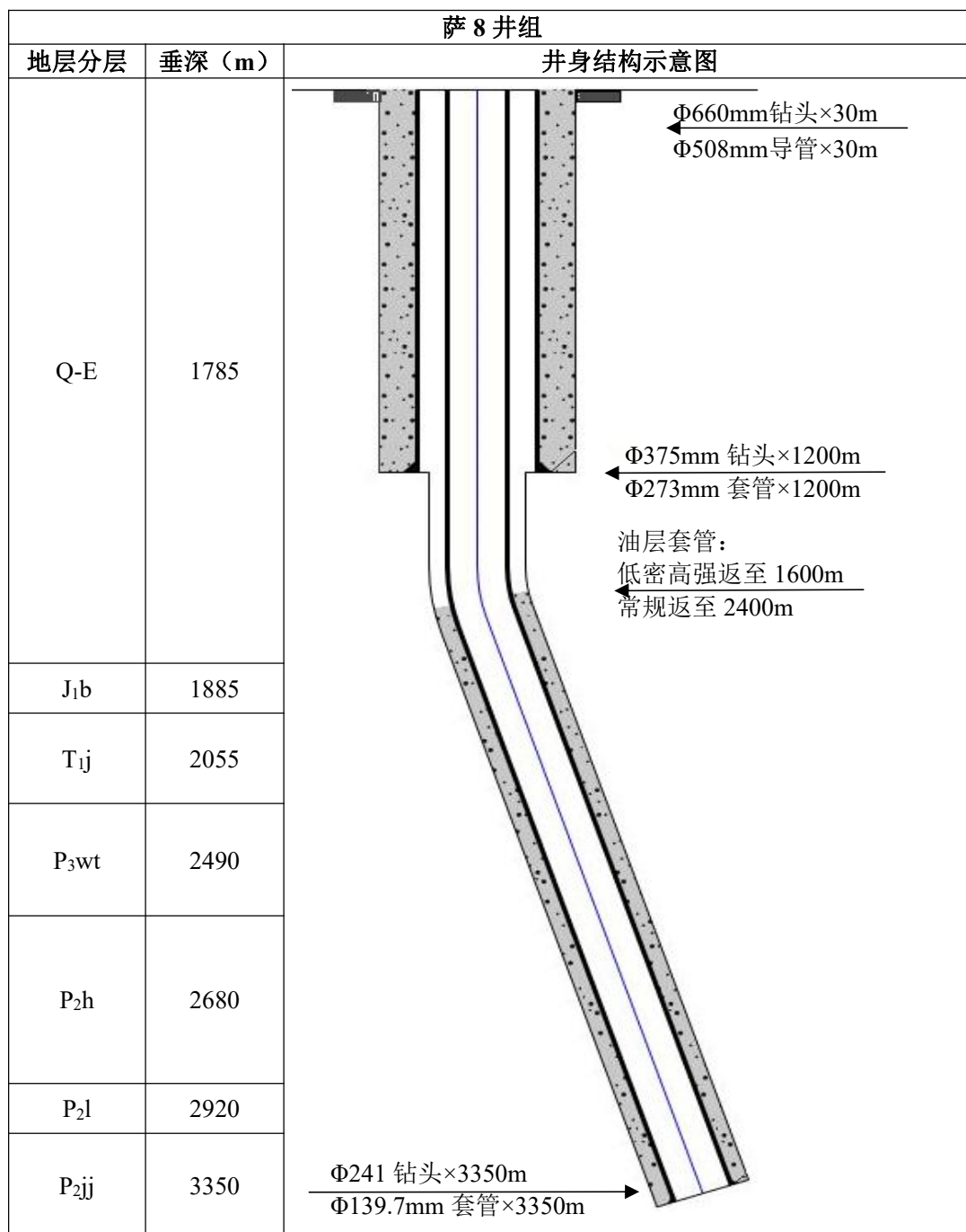
图 2-4 萨 8 井组水平井井身结构图
