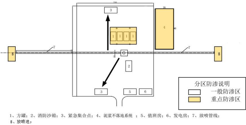
图 2-12 油气测试井场平面布置图示意图
