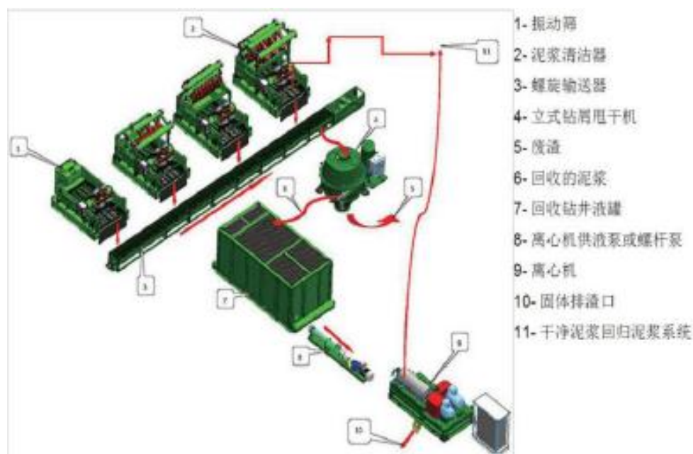
图 3.5-2 泥浆不落地处理系统工艺流程图
