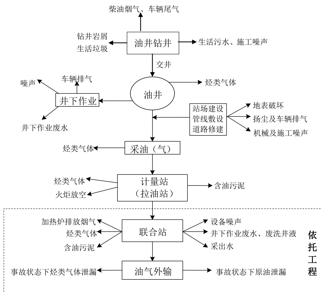
图 3.5-4 本工程开发过程污染物排放流程图
