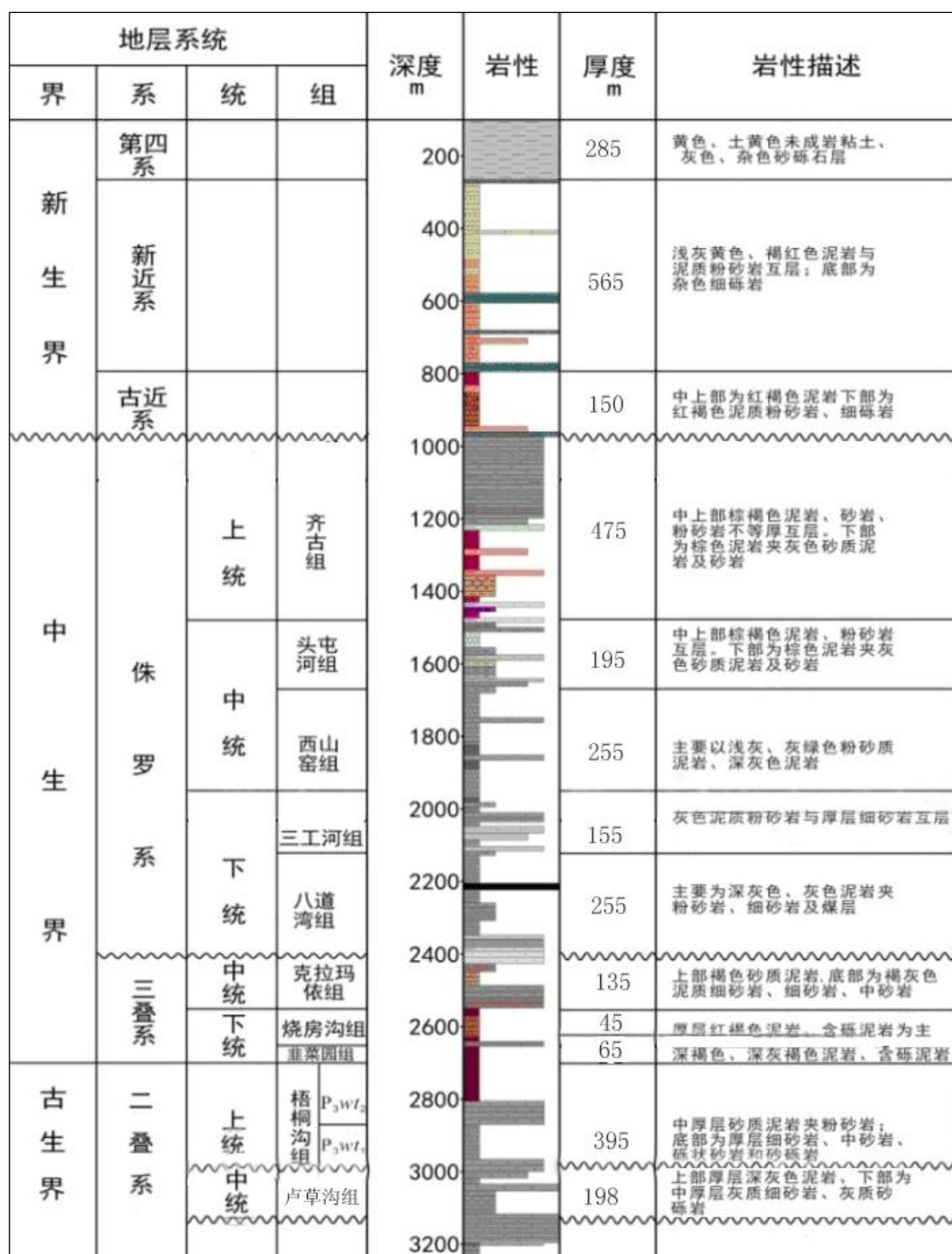
图 5.4-3 地下水水井柱状图
