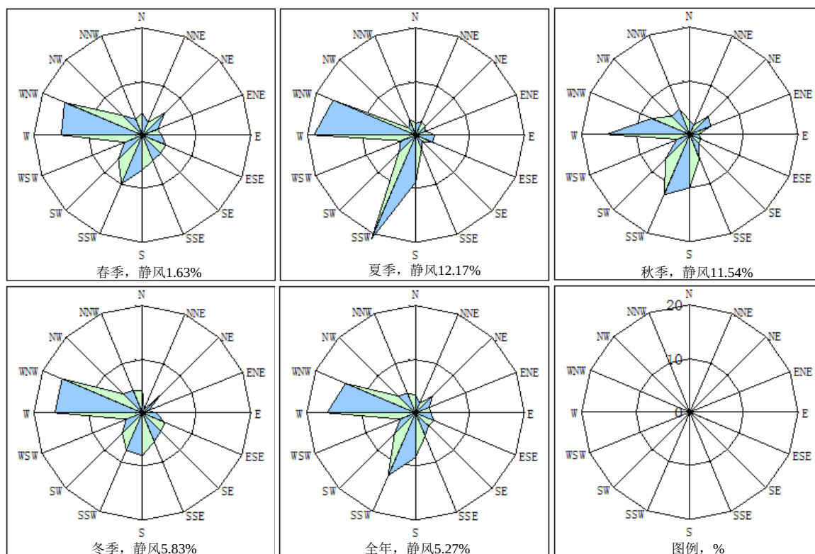
图 5.3-2 吉木萨尔县全年及各季风向频率玫瑰图
