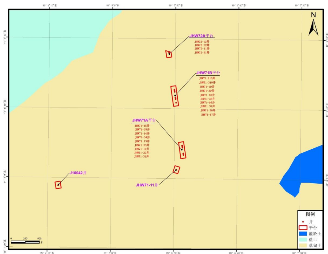
图 4.2-4 本项目所在区域土壤类型图
