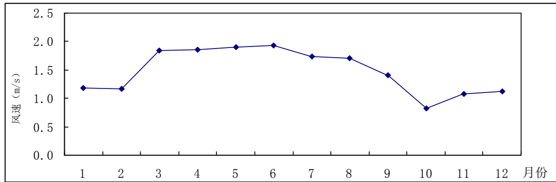
图 5.3-1 吉木萨尔县全年各月风速变化曲线
