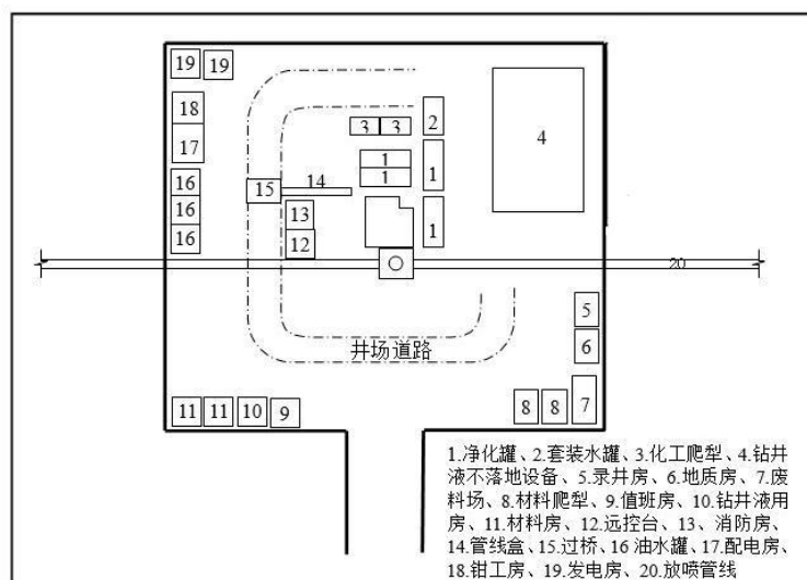
图 3.3-2 井场平面布置示意图
