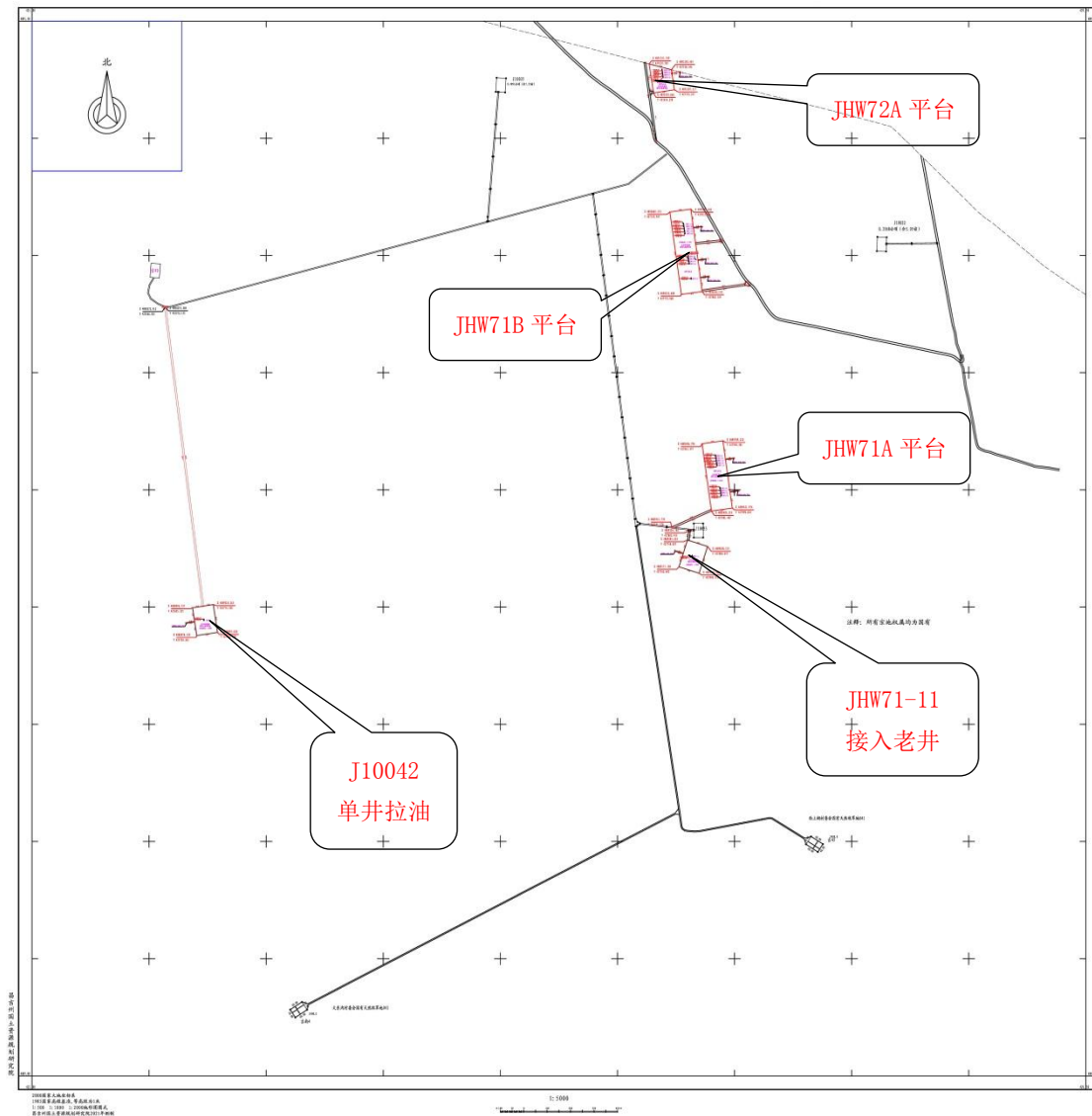
图 3.2-2 本项目总平面布置图
