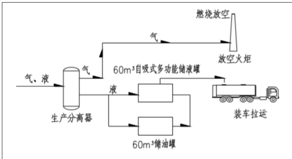
图 3.3-4 单井拉油点流程简图
