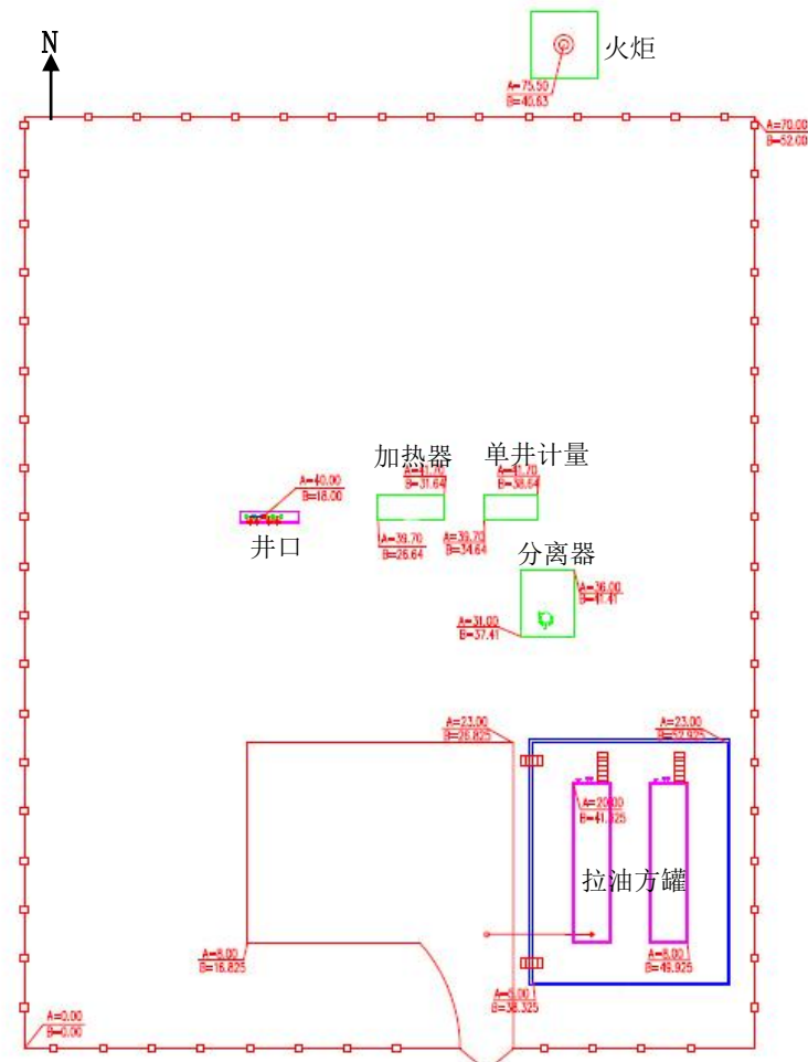
图 3.3-3 本项目单井拉油站平面布置图
