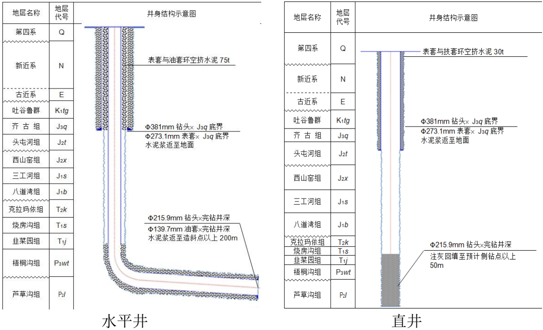
图 3.3-1 井身结构示意图
