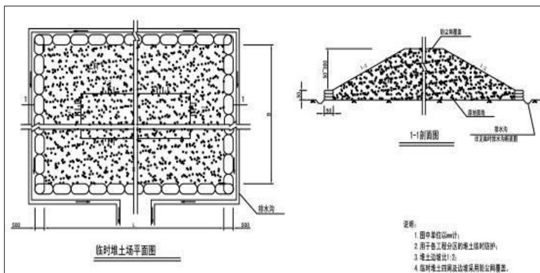
图 6.1-1 临时堆土场防护工程平面布置图
