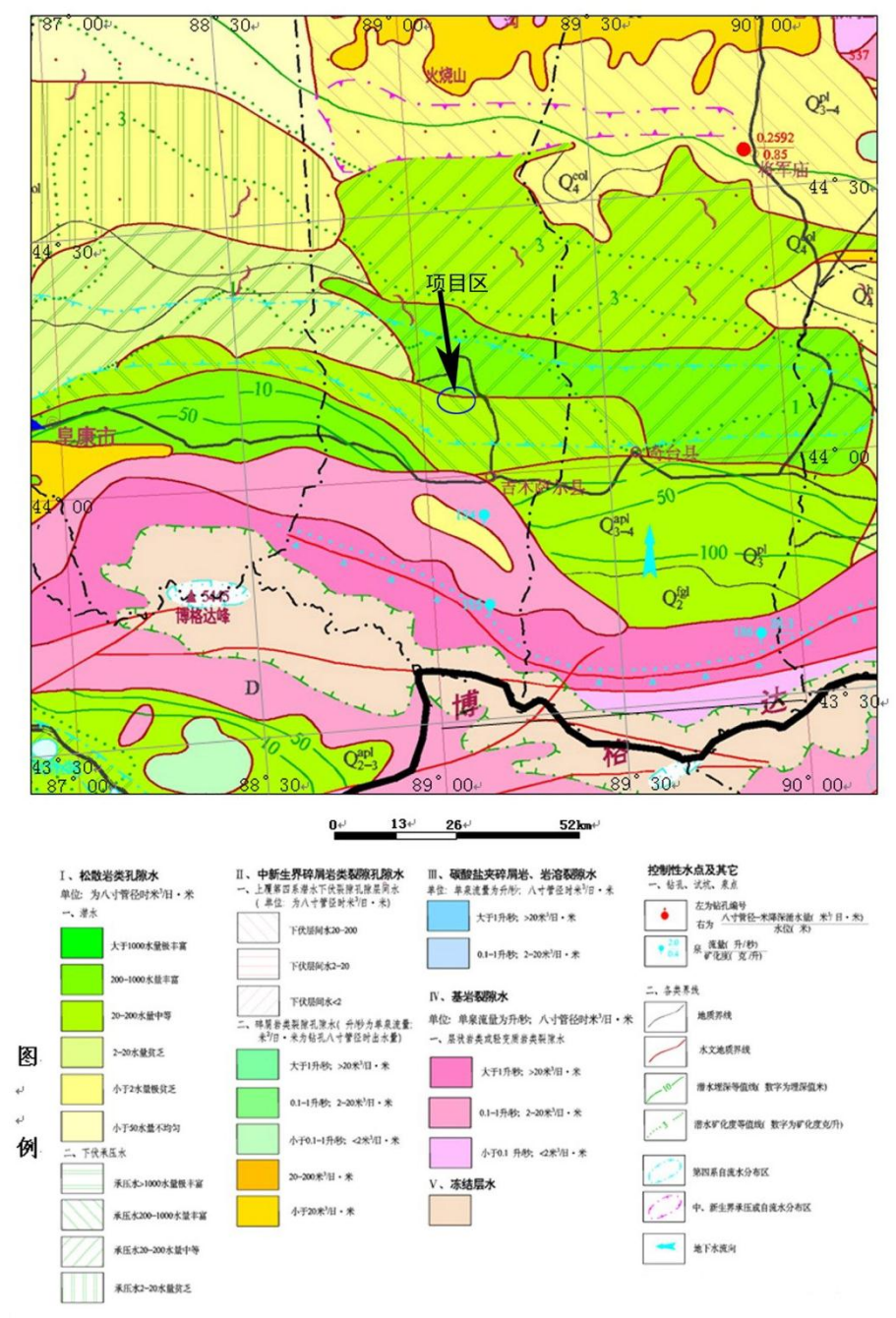
图 5.4-1 项目区水文地质图
