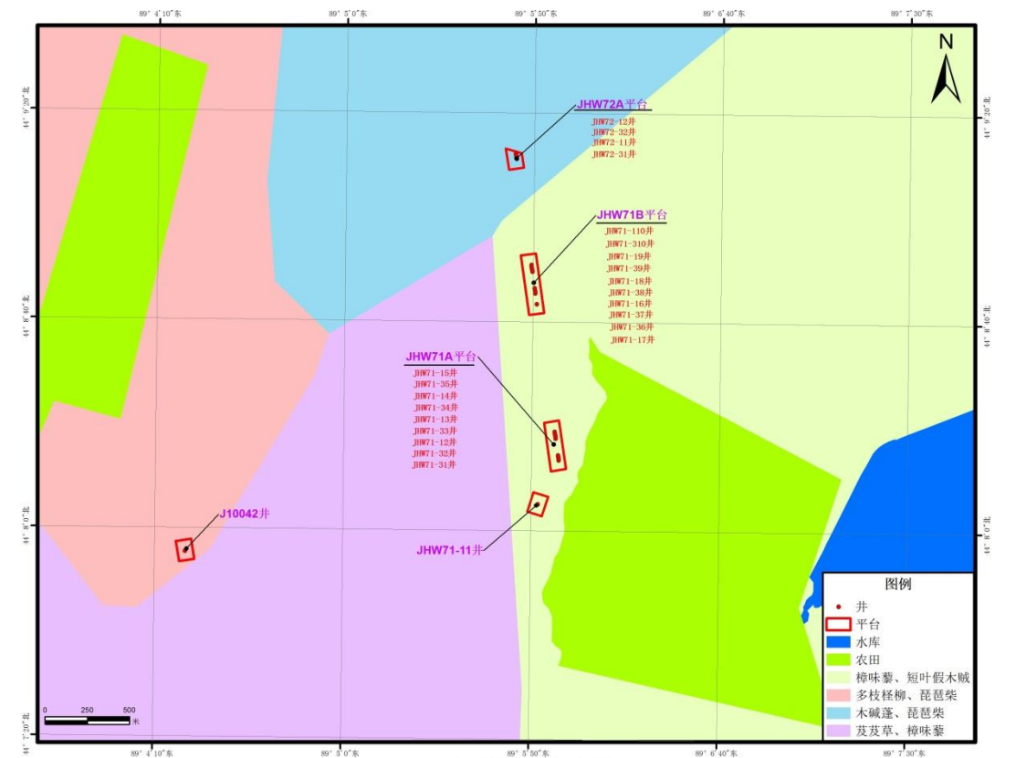
图 4.2-2 本项目所在区域植被类型图
