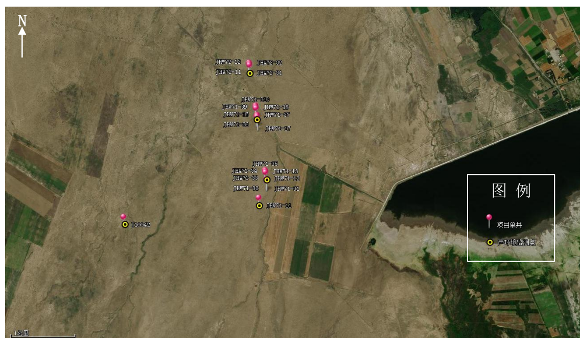
图 4.2-8 本项目声环境监测布点图
