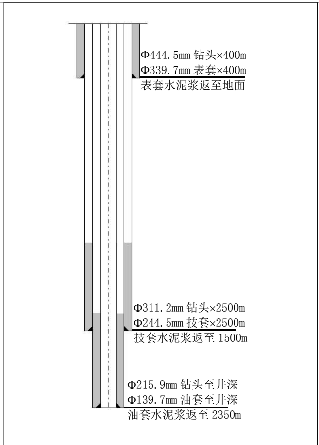
图 4 本项目井身结构示意图
