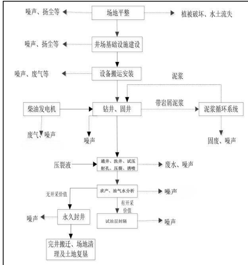
图 8 钻前工程、钻井、试油工艺流程及产污环节示意图
