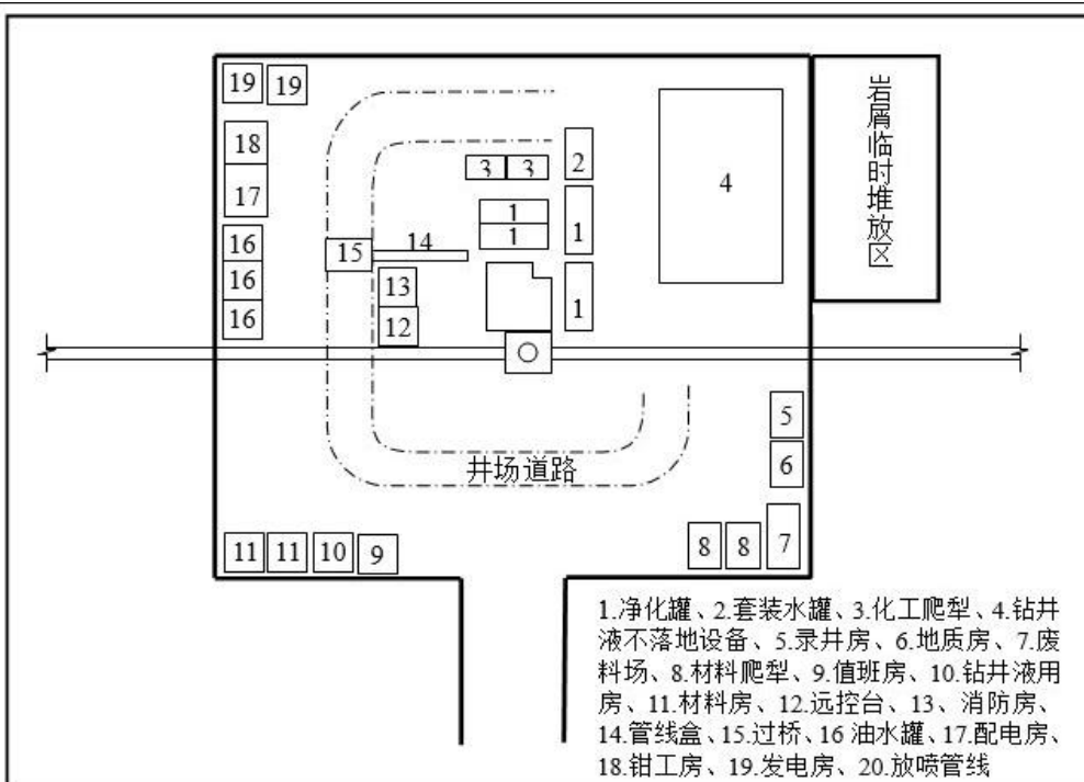
图3 井场平面布置示意图
