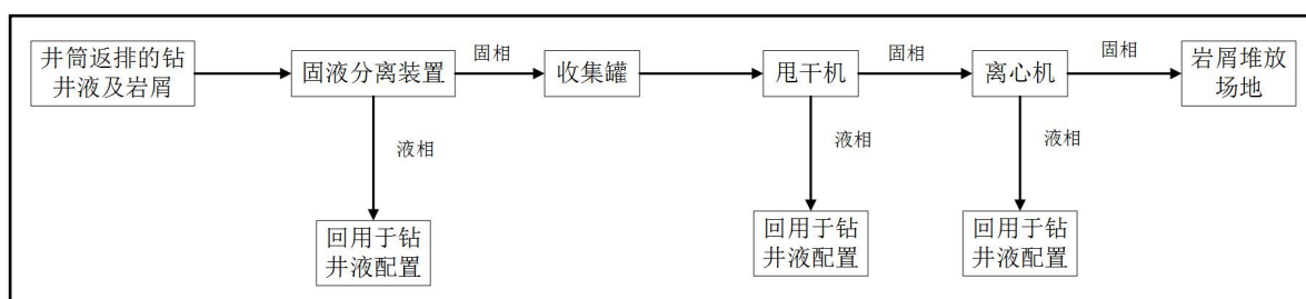
图 9 水基钻井岩屑处理工艺流程示意图
