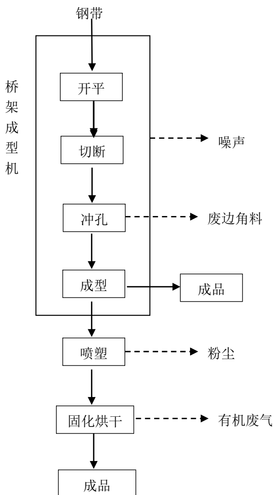
图 1 桥架生产工艺流程及产排污环节示意图
