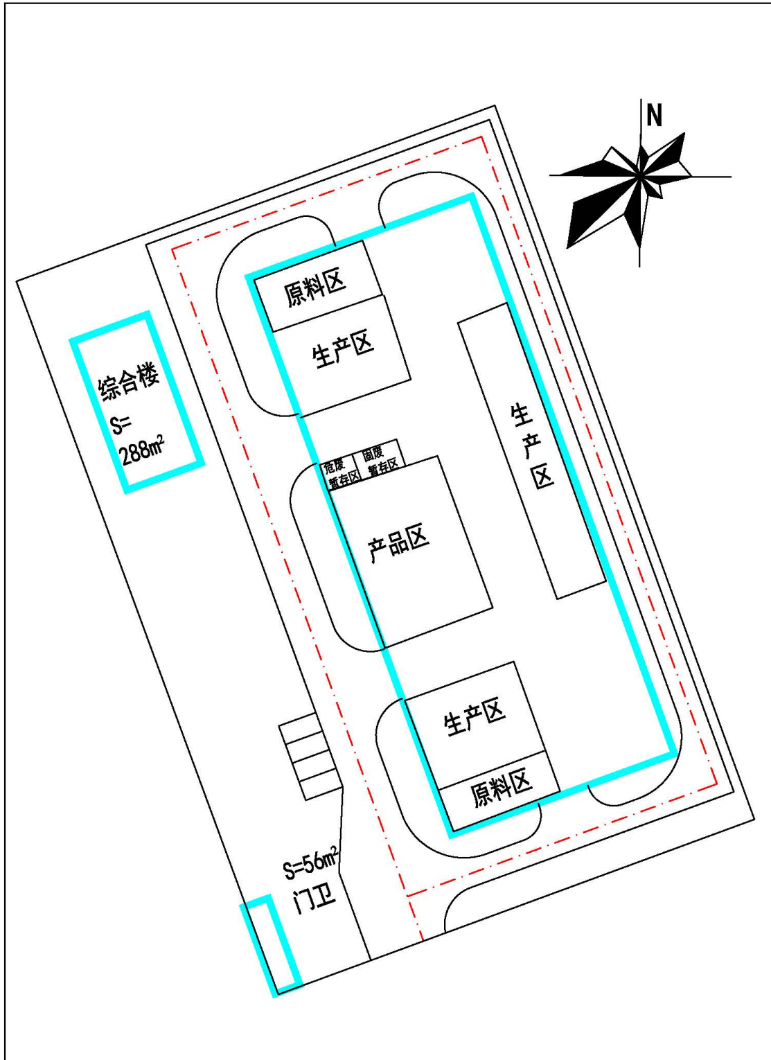
附图3 本项目厂区平面布置图
