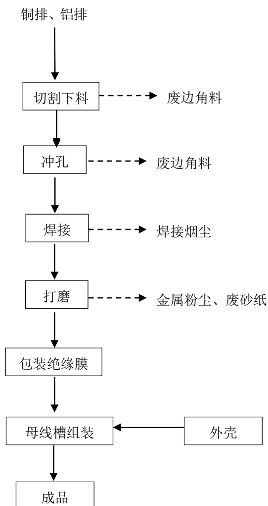
图 2 母线槽生产工艺流程图及产排污环节示意图
