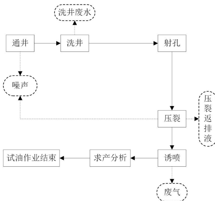
图 9 试油作业流程图
