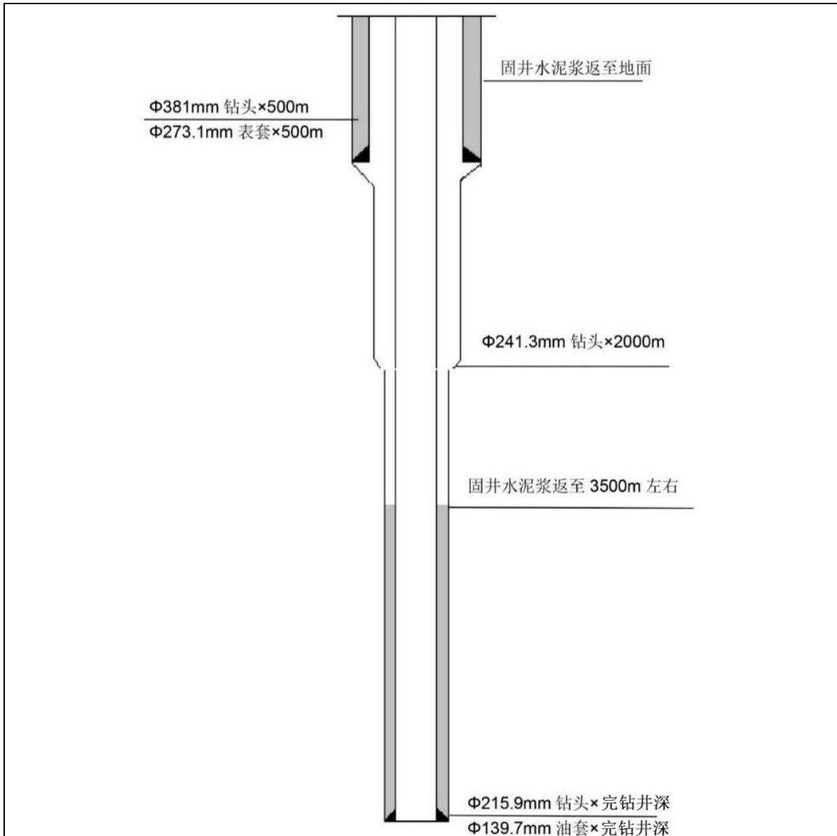
图3 井身结构示意图
