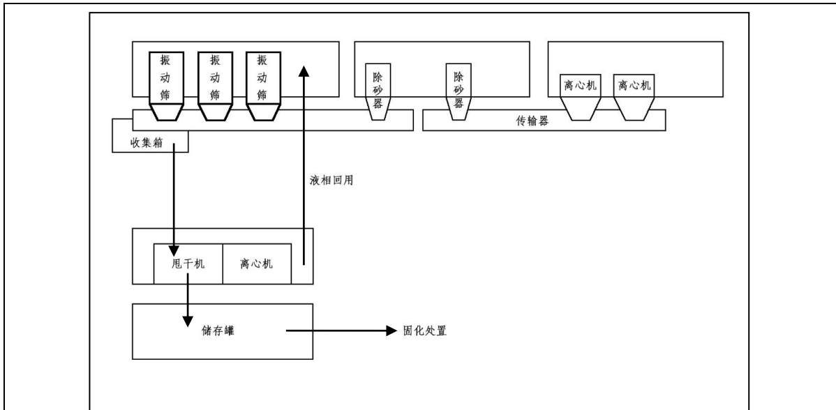
图 11 钻井液及岩屑不落地处理系统工艺流程
