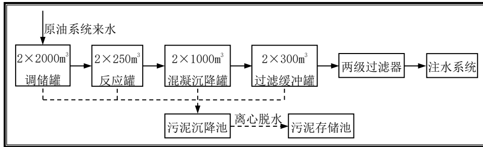
图 10 污水处理系统工艺流程图
