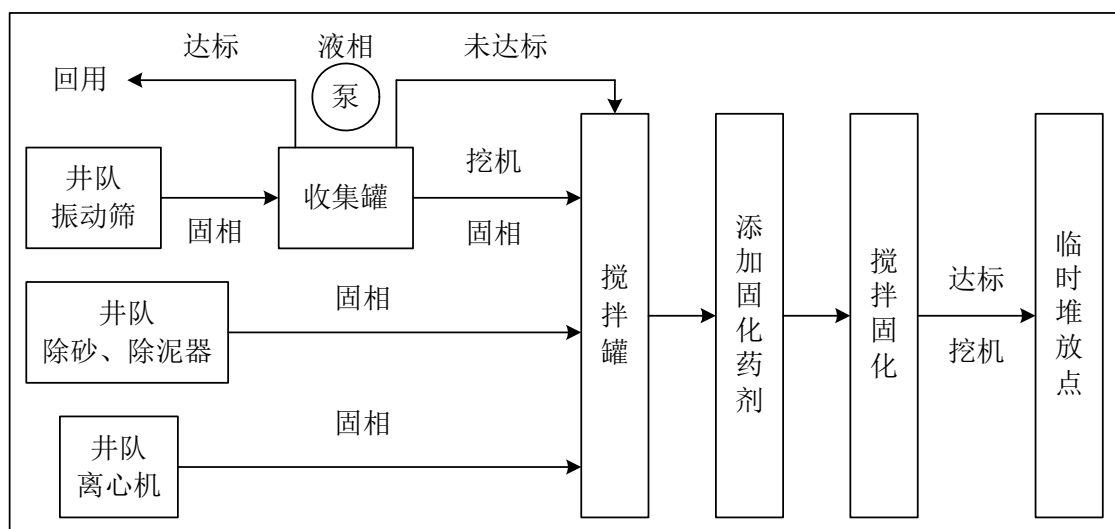
图 14 泥浆不落地装置工艺流程图
