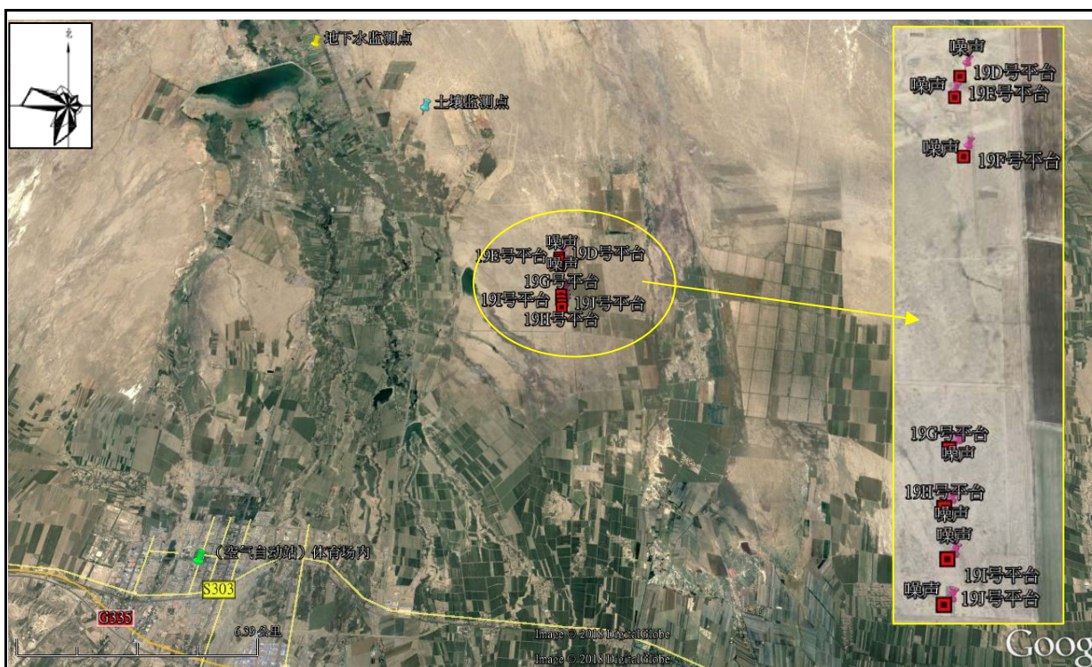
图 8 监测布点图
