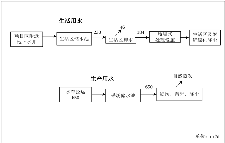
图 3-4 项目水平衡图
