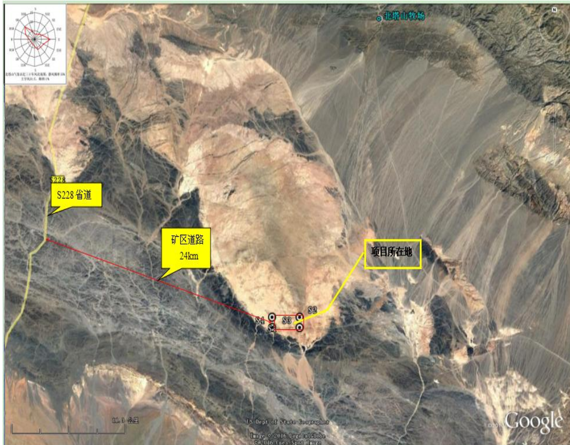
图 2.1-2 卫星遥感图
