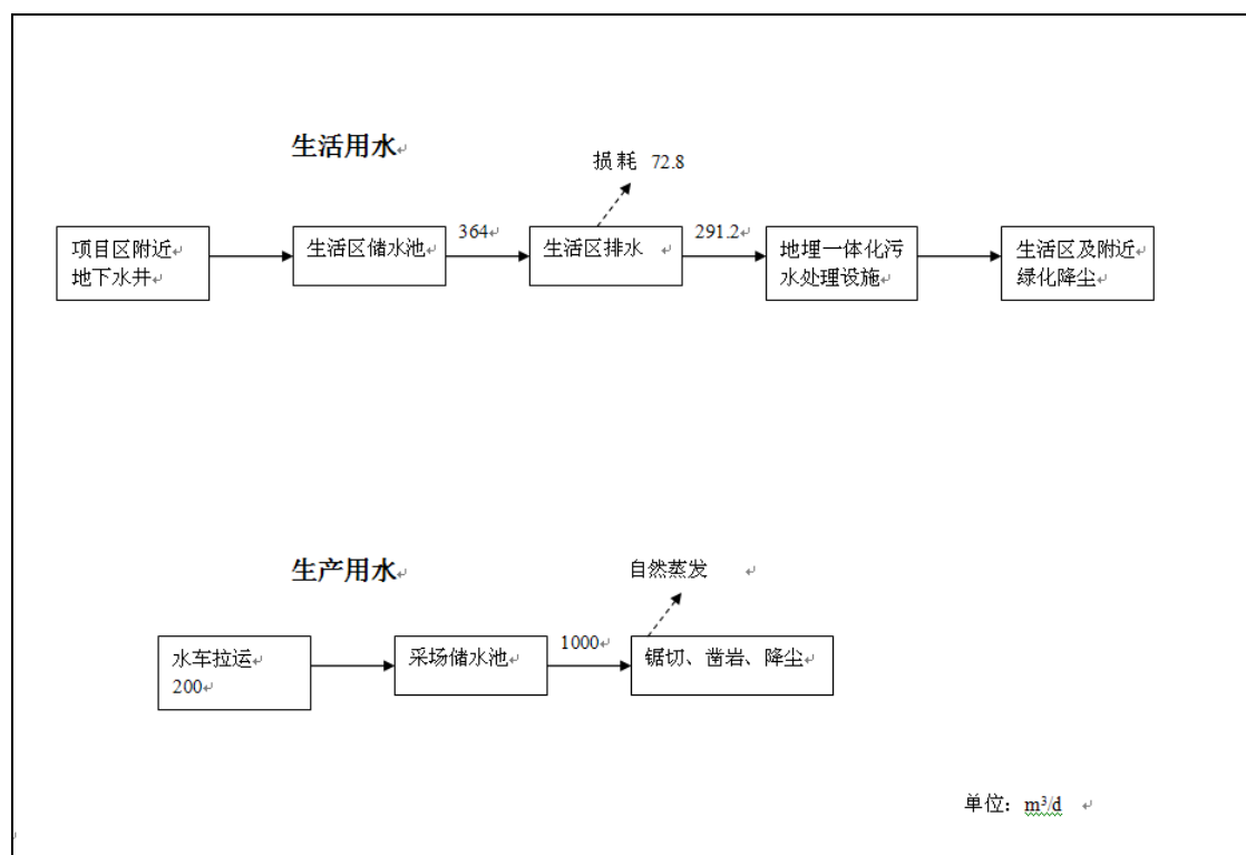
图 3.7-2 项目水平衡图
