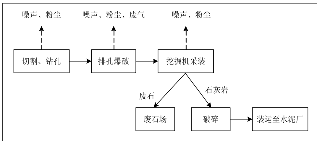
图 3-3 花岗岩开采工艺流程及产污节点示意图
