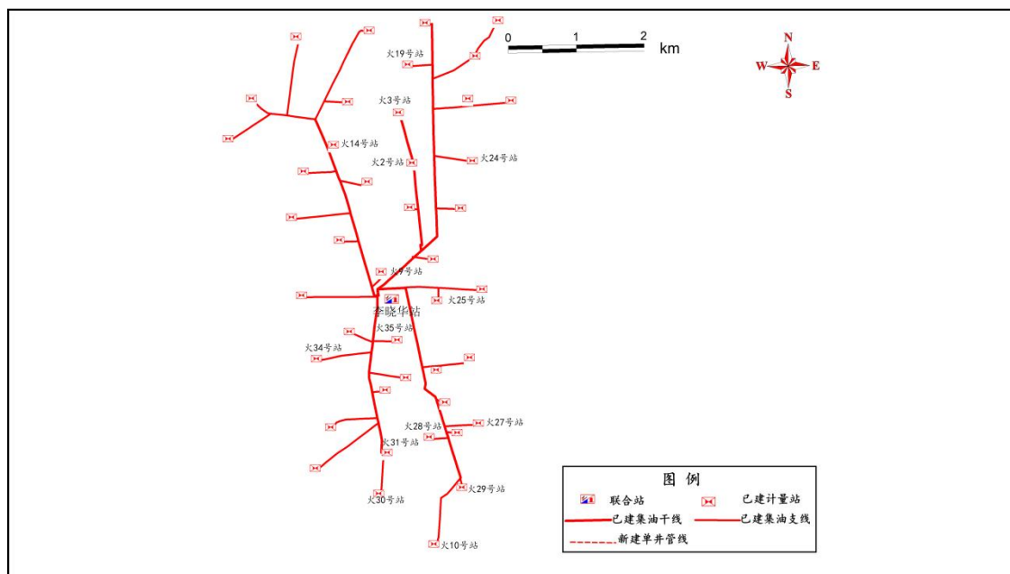
图 3.6-2 火烧山油气集输现状图
