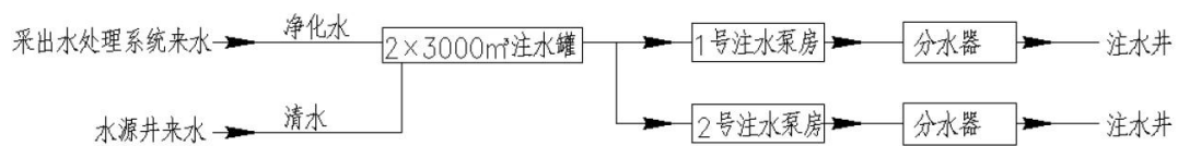
图 3.5-8 火烧山联合站注水系统流程框架图
