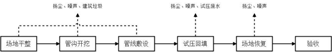
图 3.7-4 管线工程建设工艺流程及产污环节示意图
