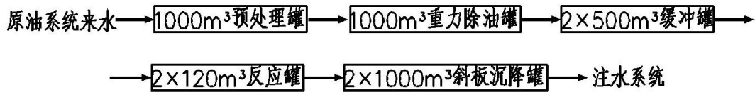
图 3.5-7 污水处理系统工艺流程图
