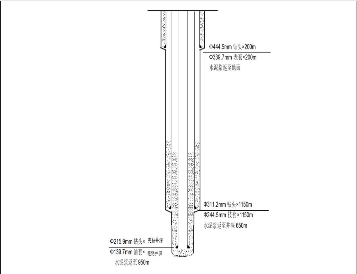
图 3.5-1 井身结构示意图
