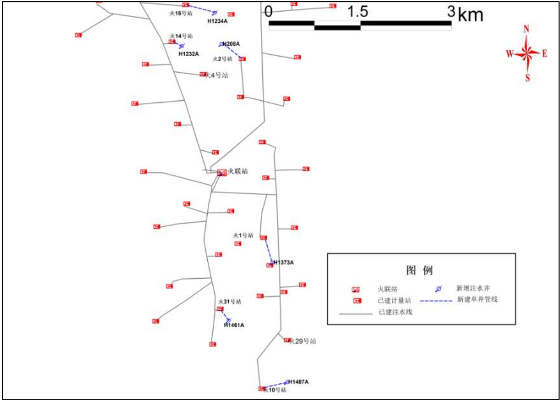
图 3.5-9 依托注水管线及本项目新建注水管线示意图
