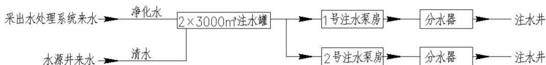
图 3.5-4 火烧山联合站注水系统流程框架图
