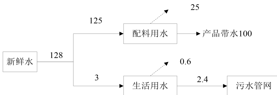
图 6 项目水平衡图（单位 m 3 /d）
