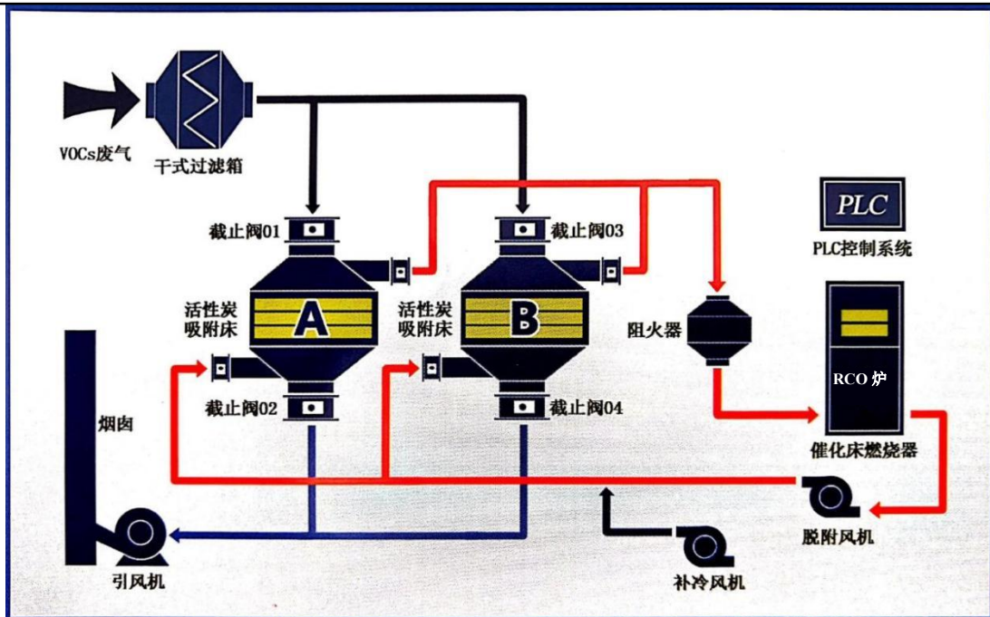
图 12 RCO 处理工艺流程图
