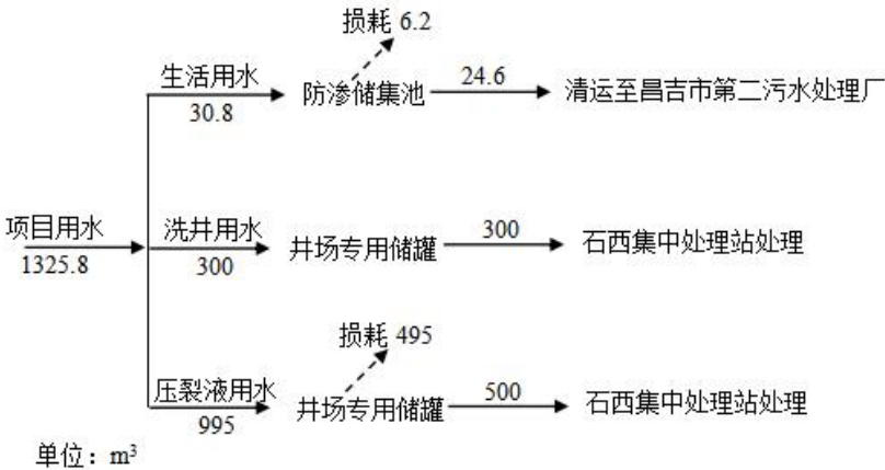
图 4-1 本项目水平衡示意图
